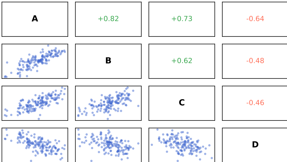
Scatterplot matrix (SPLOM)
