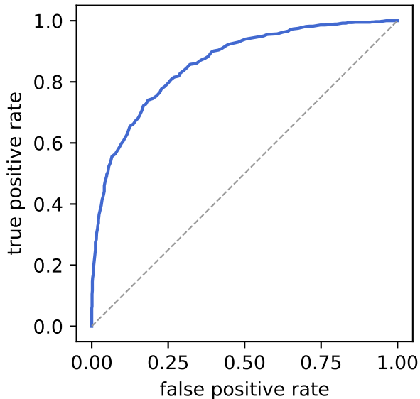
ROC (AUC = 0.86)
