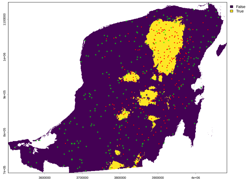
Fig. 6.6. Resultado de la función de umbralización recursiva para el 10.49% de
