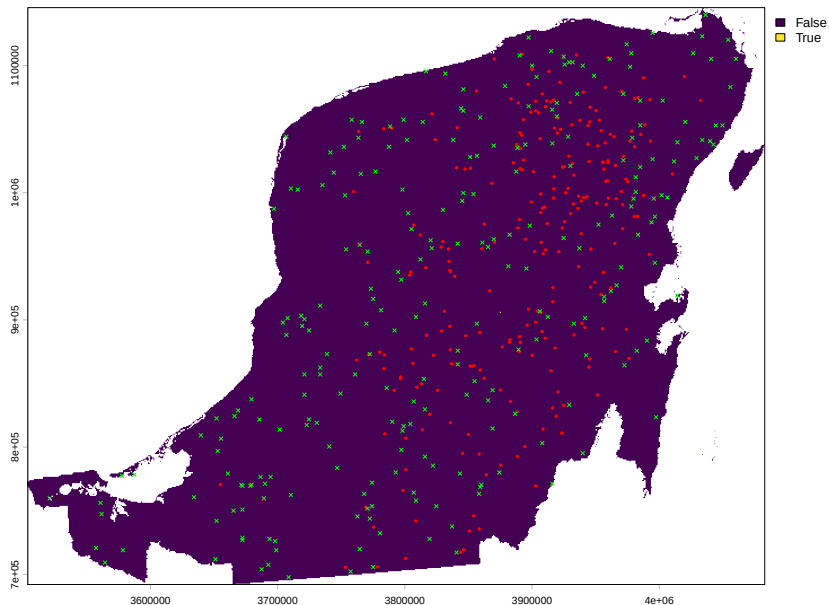
Fig. 3.6. Umbralización recursiva de la imagen de la Fig. 3.5 con un umbral de 10.
