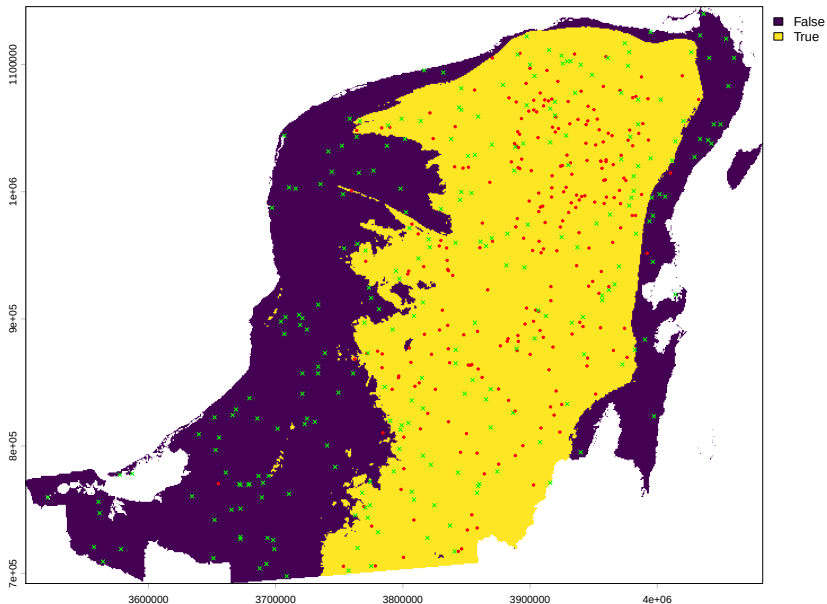
Fig. 4.6. Resultado de la función de umbralización recursiva con \alpha = 0.004 .
