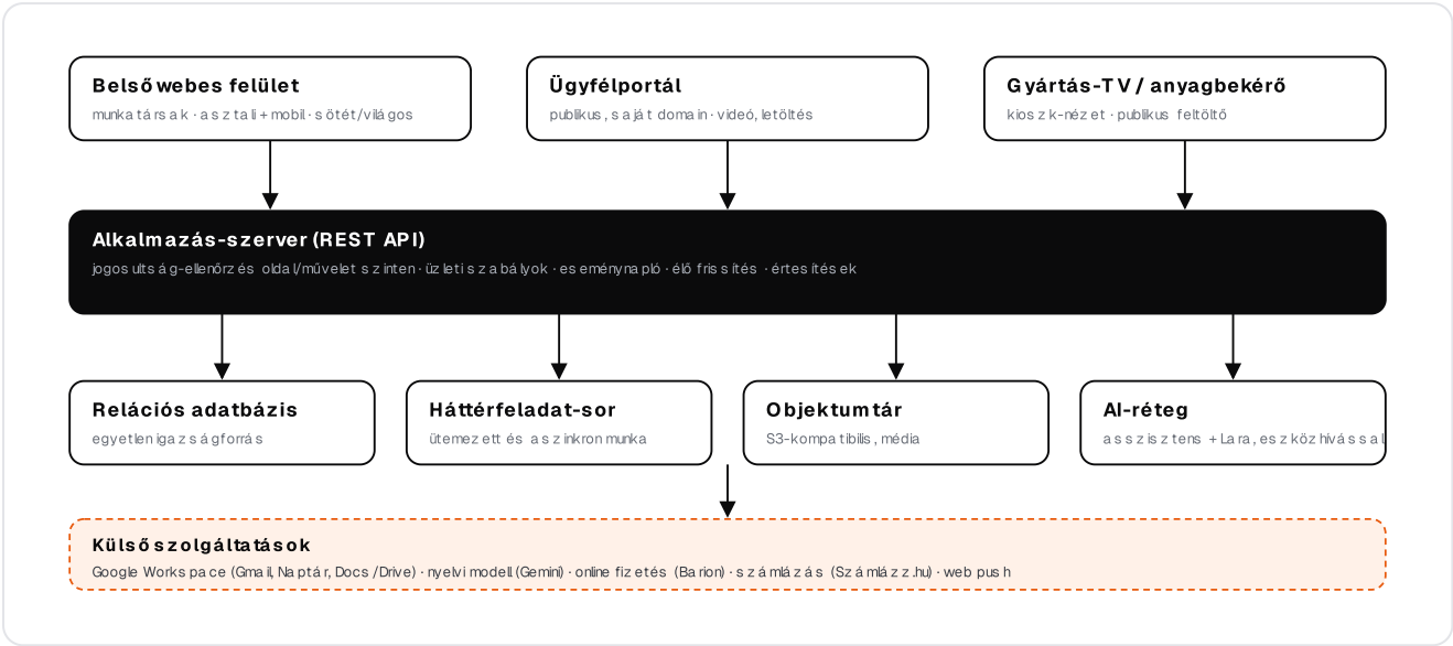
2. ábra Logikai architektúra. A konkrét technológiát az Ajánlattevő javasolja; a rétegek szétválasztása és a külső integrációk kötelezőek.
