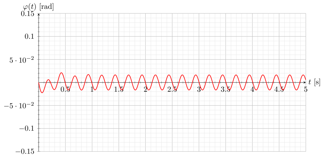
6. ábra: A rendszer gerjesztett rezgése az ütközés után
