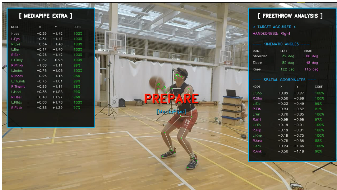
2.2. ábra. A feldolgozó rendszer által készített vizualizáció, amely valós időben mutatja az azonosított ízületi pontokat és az aktuális hajlásszögeket.
