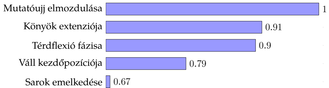
3.2. ábra. A gépi tanulási modell változóinak fontossági sorrendje (normalizált Feature Importance). A 3.2. ábra alapján látható a legmeghatározóbb tényezők rangsora.
