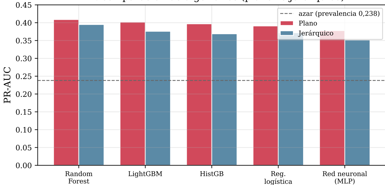
M2: comparación de algoritmos (plano vs jerárquico)
