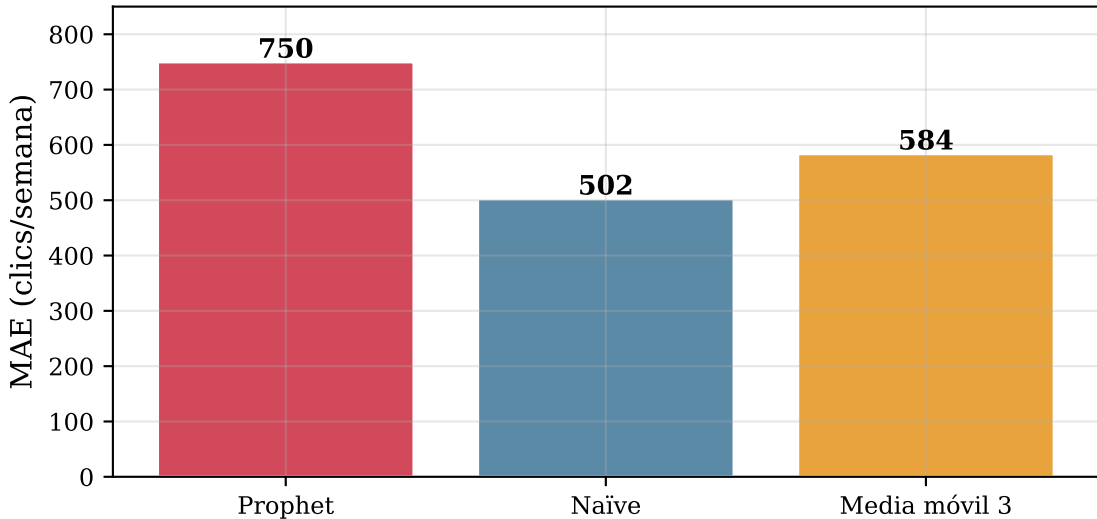
M4: error 1-paso (backtest rolling) — menor es mejor
