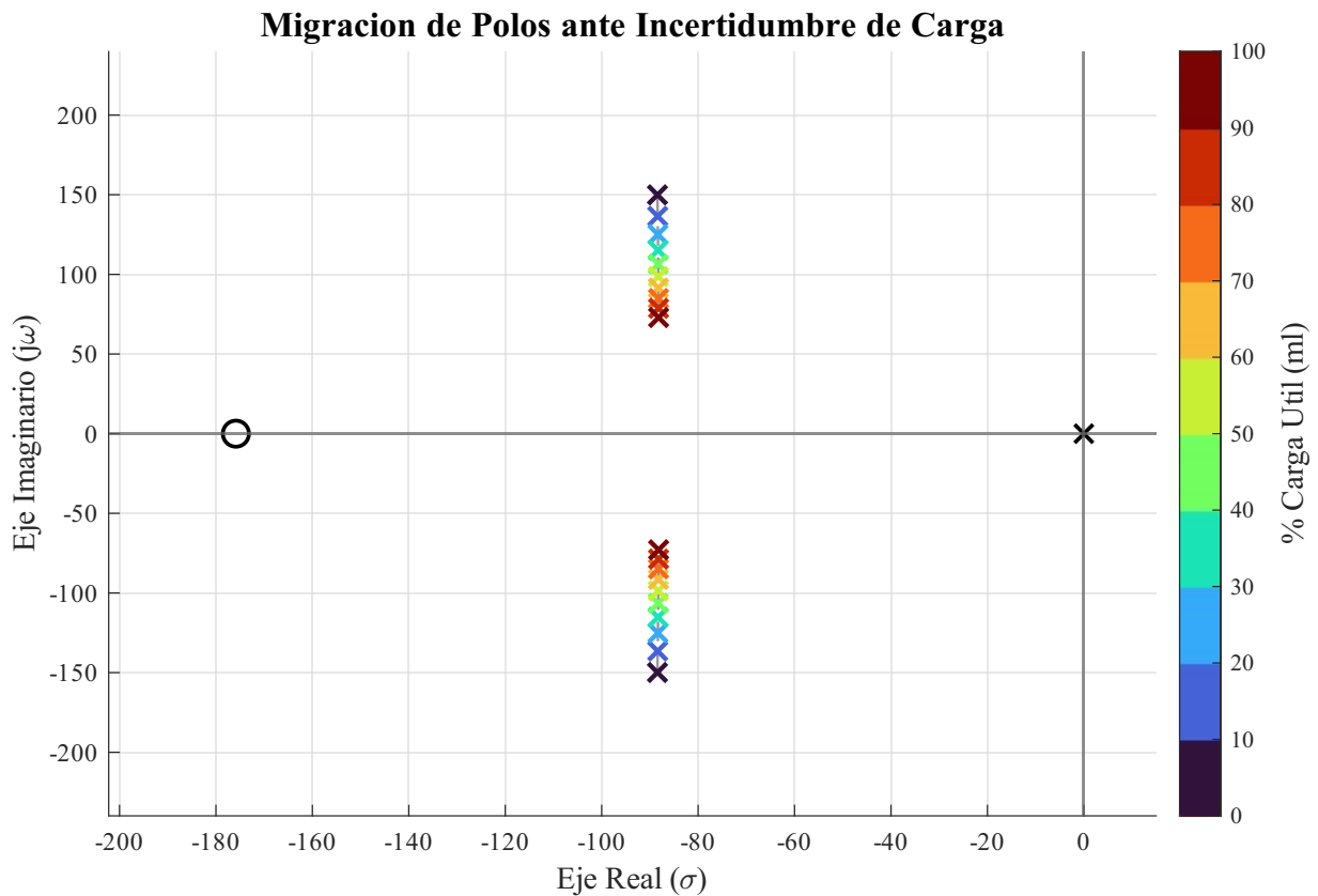
Figura 12: Migración de los polos electromecánicos conjugados p_{2,3} en el plano s ante el aumento progresivo de la masa de carga útil m_l (desde 0 % a 100 % de carga máxima).
