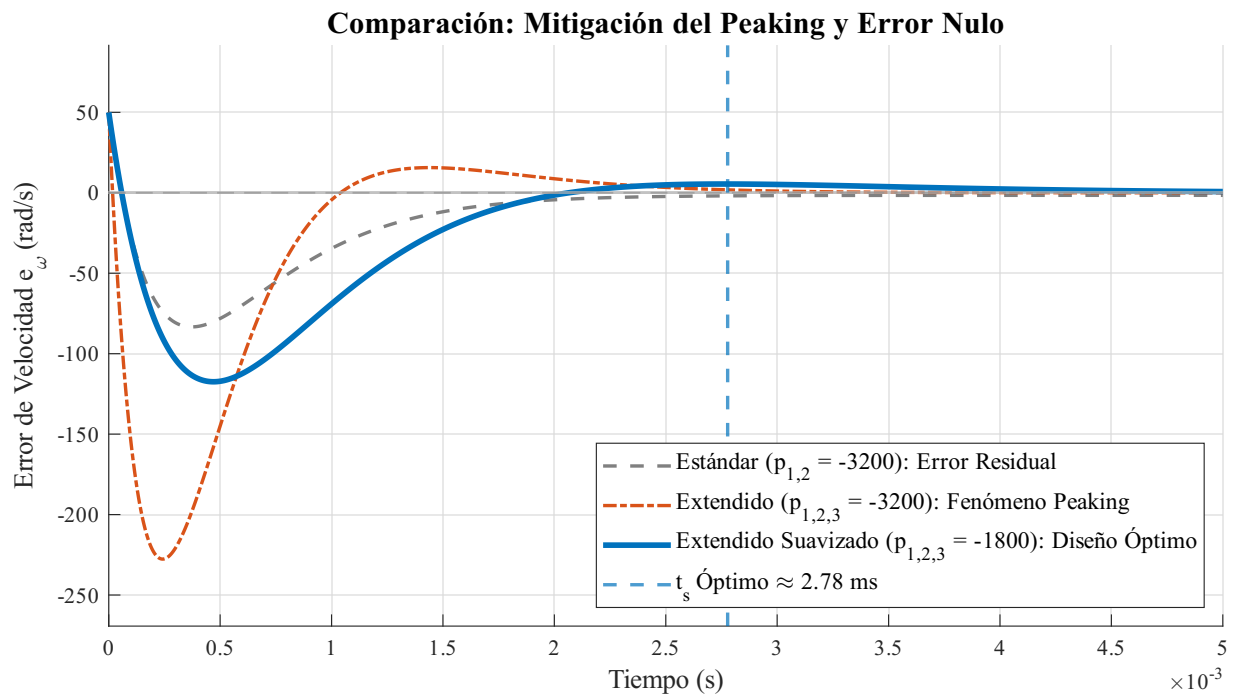
Figura 69: Comparativa global de la dinámica del error aislada. El diseño óptimo (suavizado a -1800 rad/s) encuentra el equilibrio ideal entre velocidad de convergencia, atenuación del peaking y error nulo.
