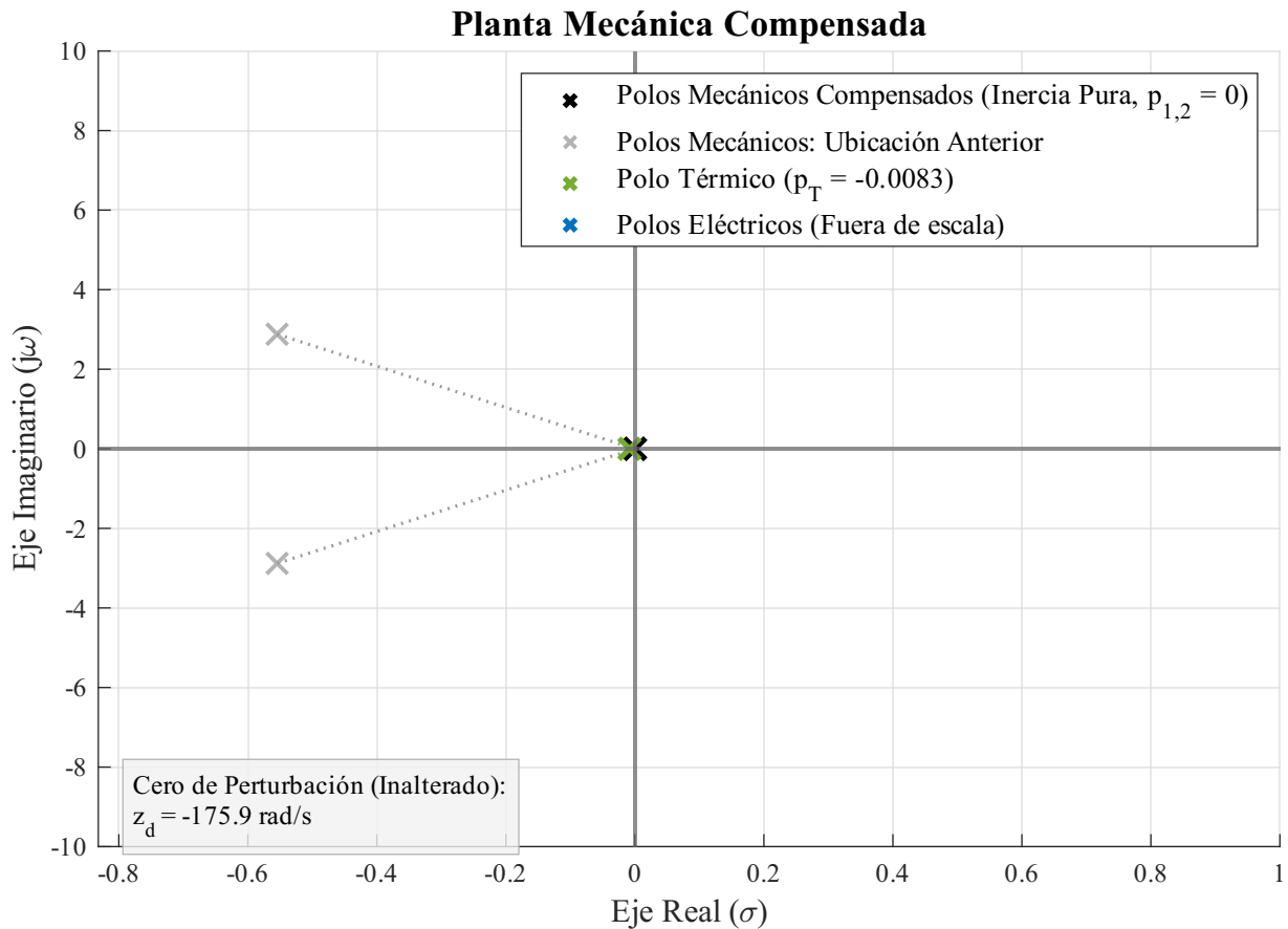
Figura 49: Mapa de polos mecánicos tras aplicar el Modulador de Torque con compensación de fricción y gravedad. Los polos convergen al origen, configurando una planta integradora ideal ( 1/J_{eq}s ).
