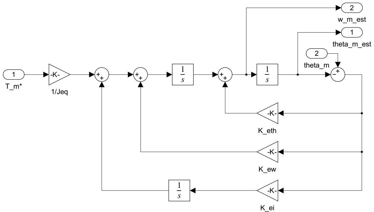
Figura 67: Diagrama de bloques del Observador de Estado Extendido en Simulink. La adición del estado integrador ( K_{ei}/s ) elimina el error de estimación estacionario ante torques de carga desconocidos.
