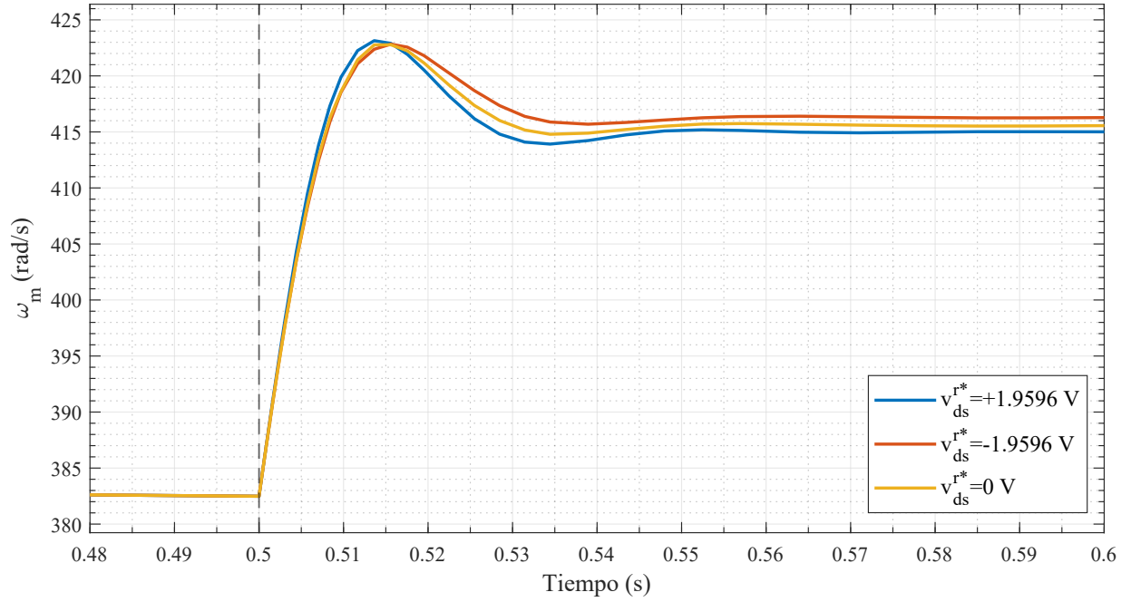
Figura 43: Velocidad angular del modelo no lineal ante reforzamiento y debilitamiento de campo.
