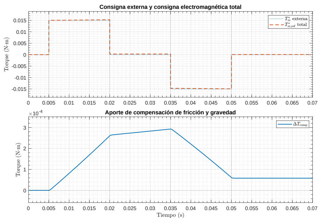
Figura 52: Consigna externa, referencia electromagnética total y aporte de la compensación de fricción y gravedad.
