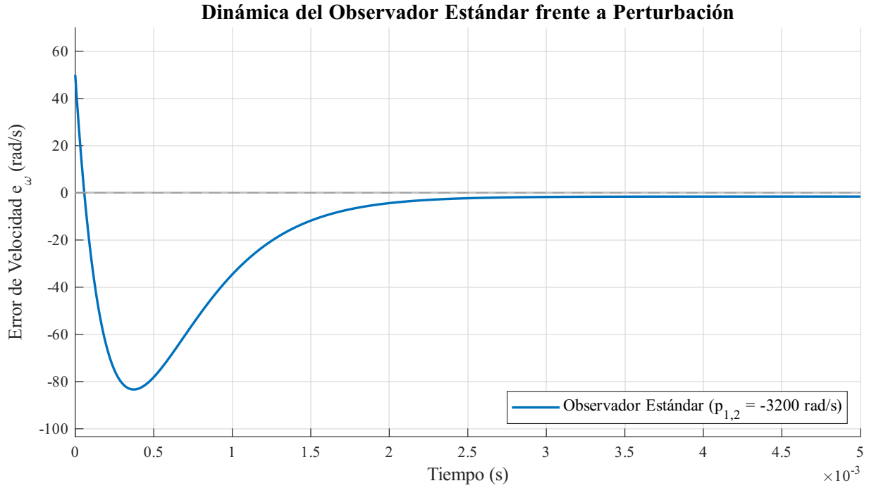
Figura 66: Dinámica del error de estimación del observador estándar de orden 2. Ante una perturbación de torque activa, el sistema presenta un error de velocidad residual.
