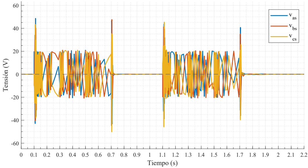
Figura 25: Tensiones estatóricas de fase v_a(t) , v_b(t) y v_c(t) , expresadas en coordenadas abc .
