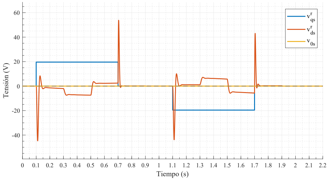
Figura 26: Tensiones estatóricas v_{qs}^r(t) , v_{ds}^r(t) y v_{0s}(t) , expresadas en coordenadas virtuales qd0 .
