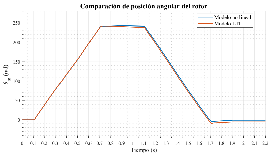
Figura 28: Comparación de la posición angular del rotor \theta_m(t) obtenida con los modelos no lineal y LTI.
