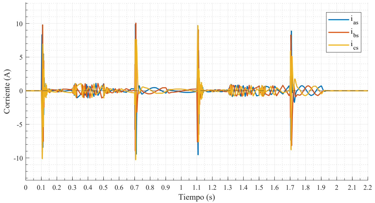
Figura 23: Corrientes estáticas de fase i_a(t) , i_b(t) e i_c(t) , expresadas en coordenadas abc .
