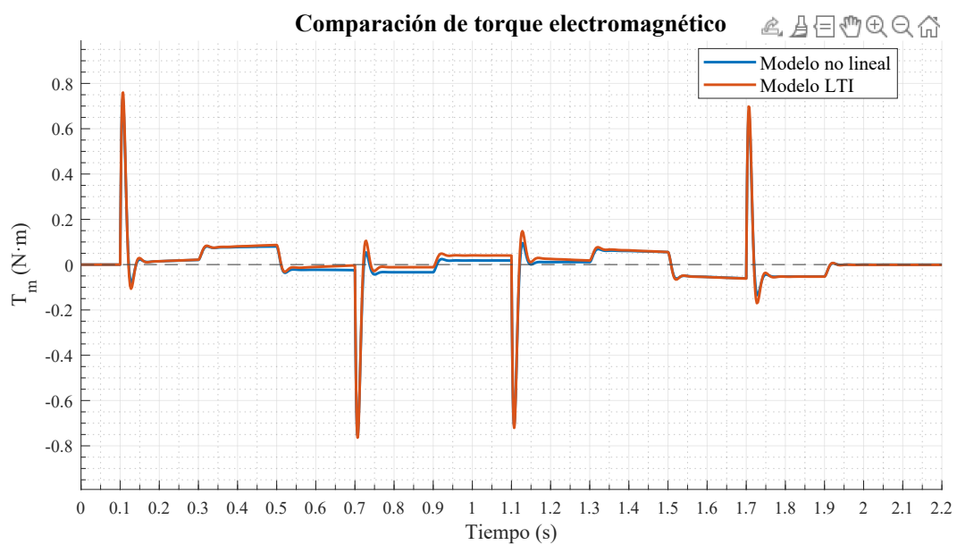
Figura 30: Comparación del torque electromagnético del motor T_m(t) obtenido con los modelos no lineal y LTI.
