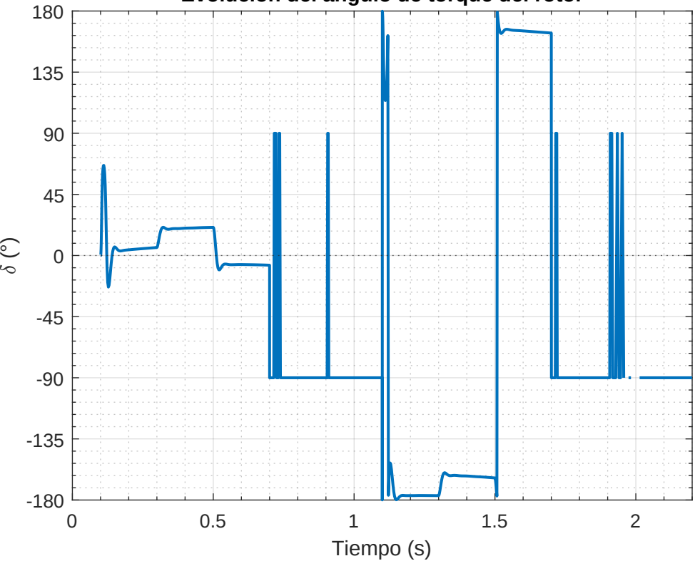
Evolución del ángulo de torque del rotor
