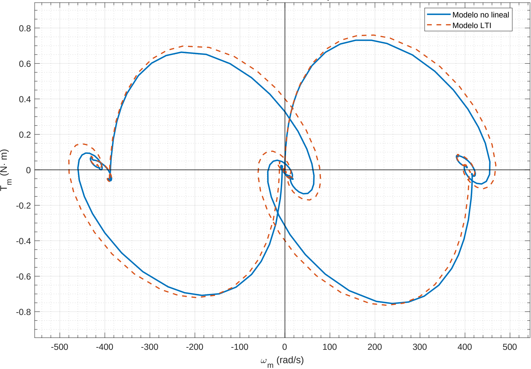
Comparación de trayectorias torque-velocidad
