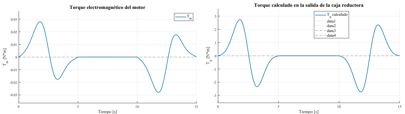
(a) Torque electromagnético desarrollado por el motor.
