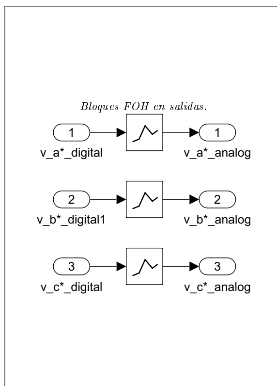
Figura 100: Conversores DAC implementados mediante retención de primer orden (FOH).
