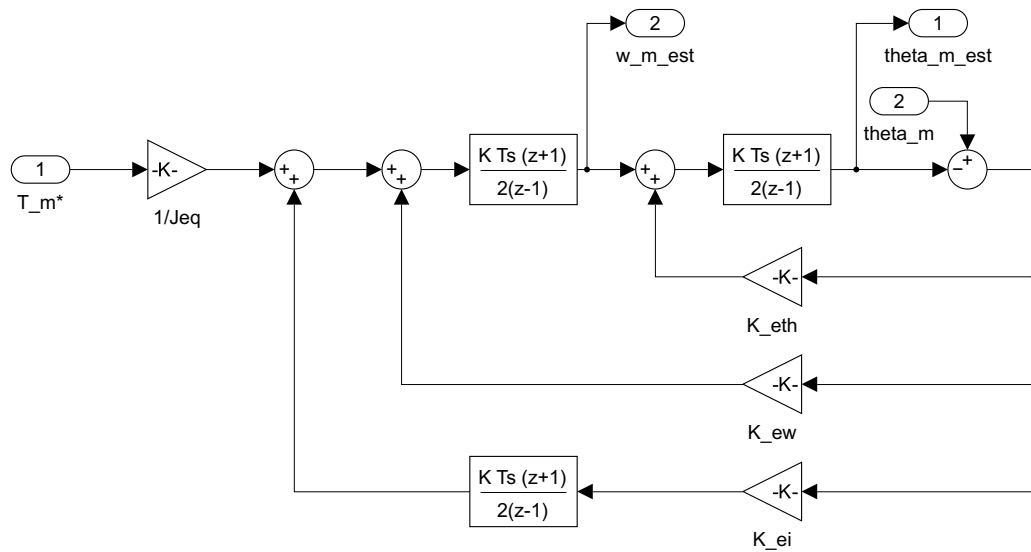
Figura 102: Topología discreta del Observador Reducido de Estado, forzando la digitalización de sus entradas y su dinámica interna mediante el método bilineal.
