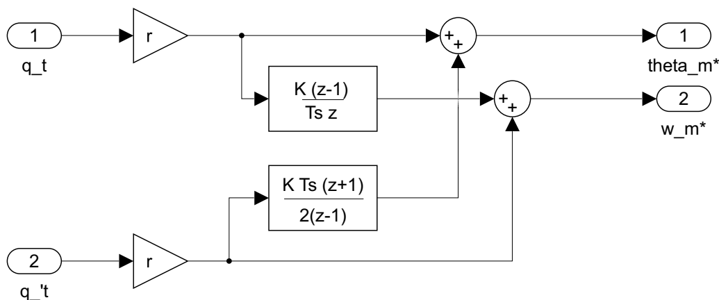
Figura 103: Implementación en tiempo discreto de la Interfaz de Referencia (Set-Point).
