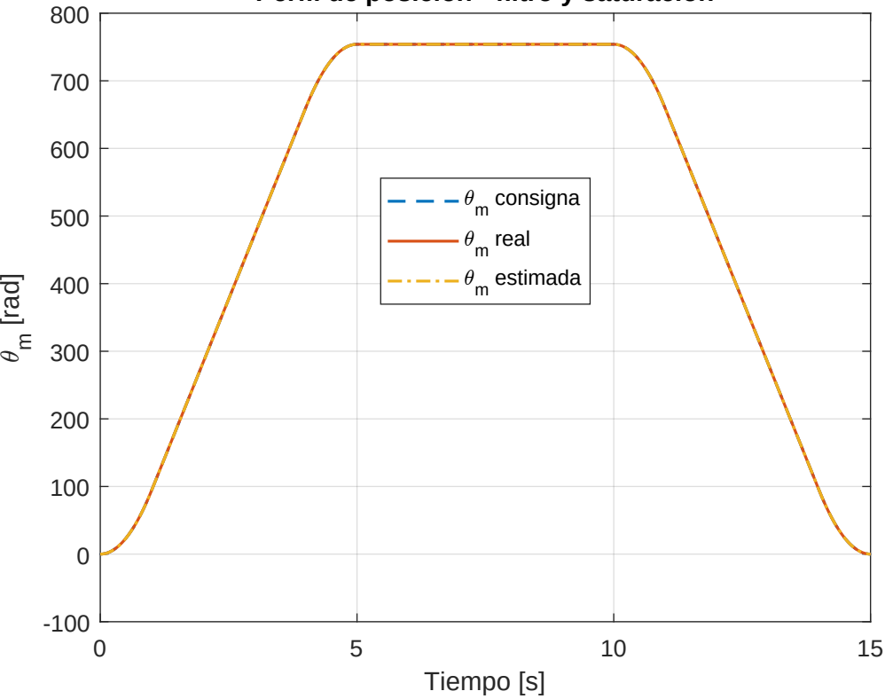
Perfil de posición - filtro y saturación
