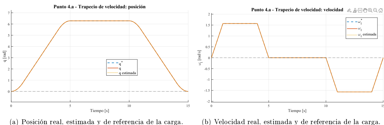
Figura 73: Seguimiento de posición y velocidad para la consigna trapezoidal de velocidad.
