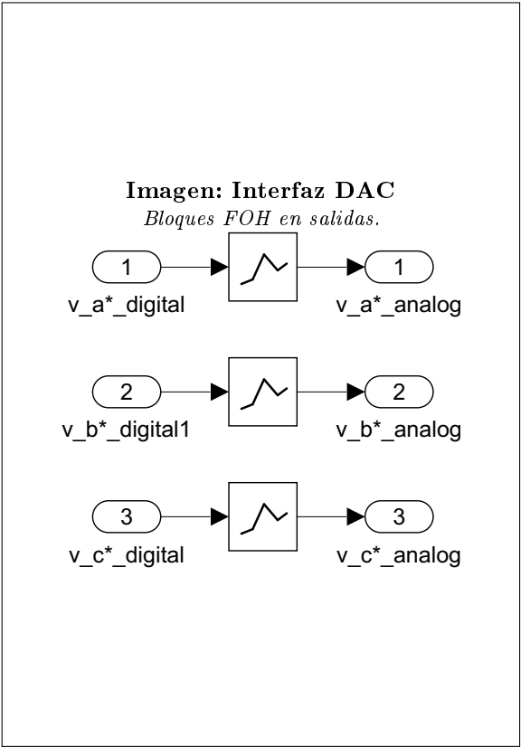
Figura 89: Conversores DAC implementados mediante retención de primer orden (FOH).
