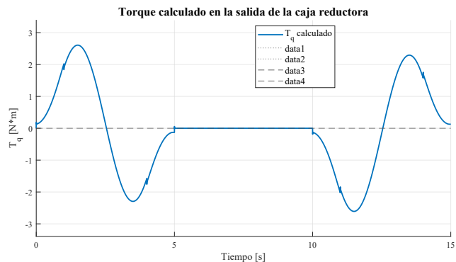
(b) Torque calculado en la salida de la caja reductora.
