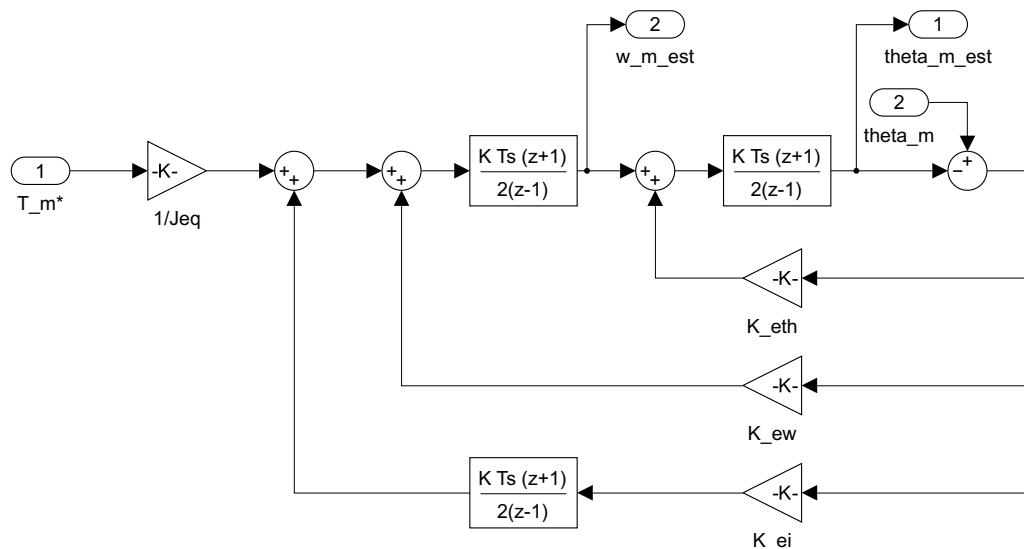
Figura 91: Topología discreta del Observador Reducido de Estado, forzando la digitalización de sus entradas y su dinámica interna mediante el método bilineal.
