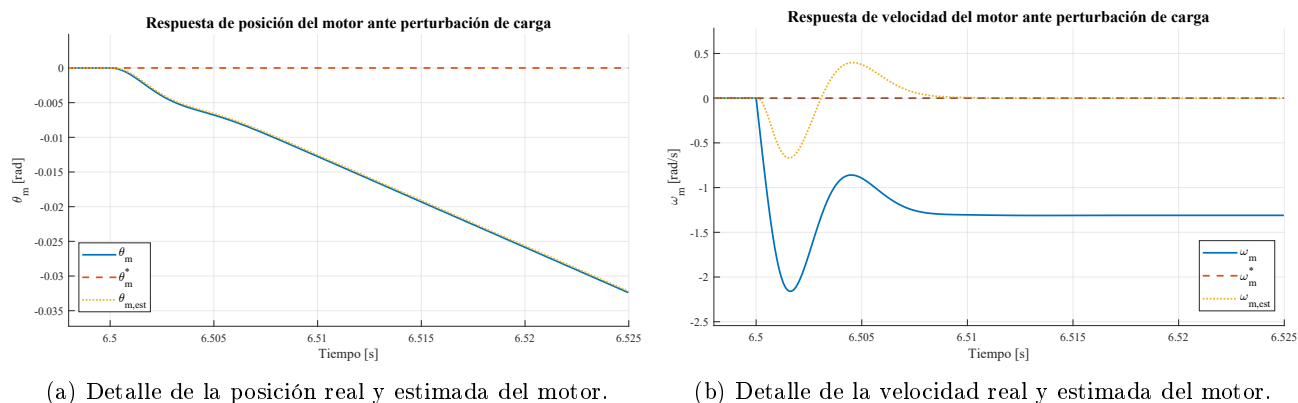
Figura 72: Detalle de la respuesta del motor en el instante de aplicación de la perturbación para el caso nominal.
