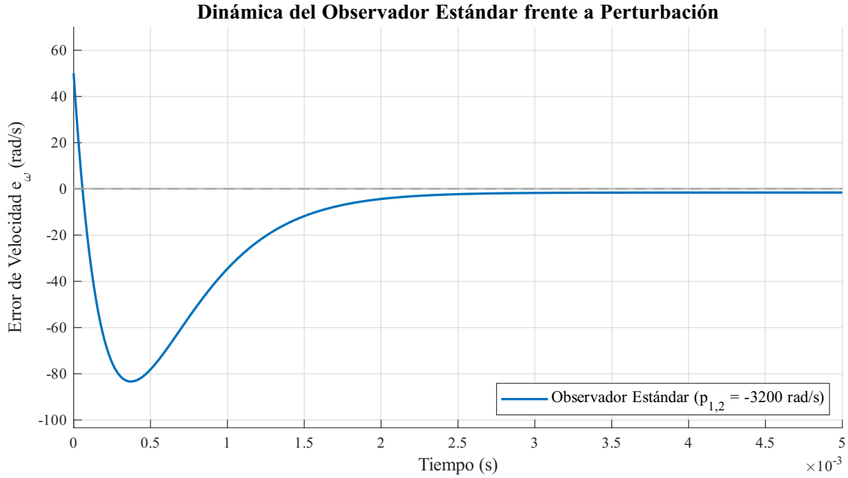
Figura 81: Dinámica del error de estimación del observador estándar de orden 2. Ante una perturbación de torque activa, el sistema presenta un error de velocidad residual.
