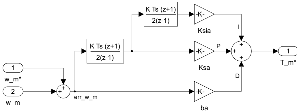
Figura 90: Estructura del Controlador PID en dominio discreto, reemplazando los integradores continuos por equivalentes trapezoidales de Tustin con T_s = 0,0001 s.
