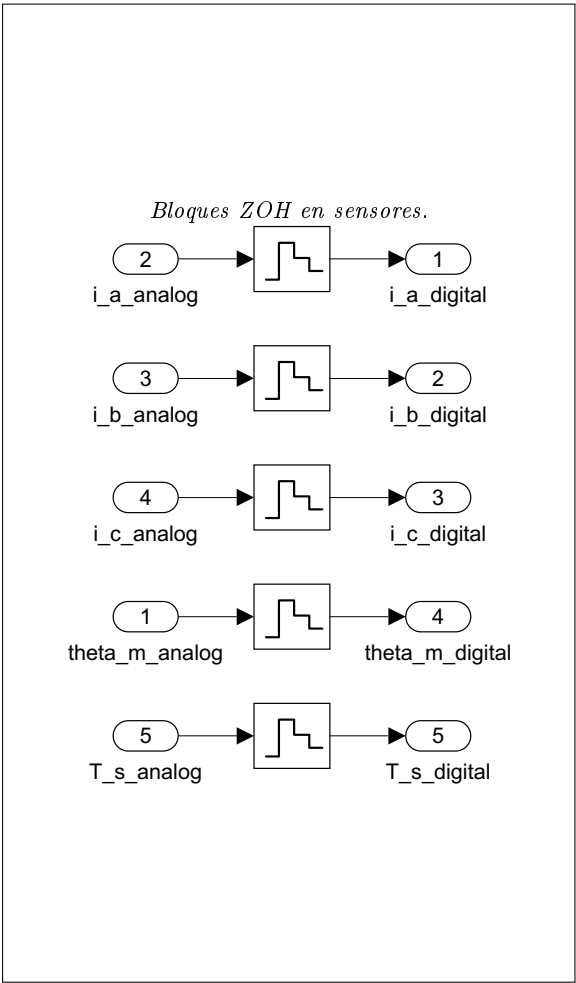
Figura 88: Conversores ADC implementados mediante retención de orden cero (ZOH).
