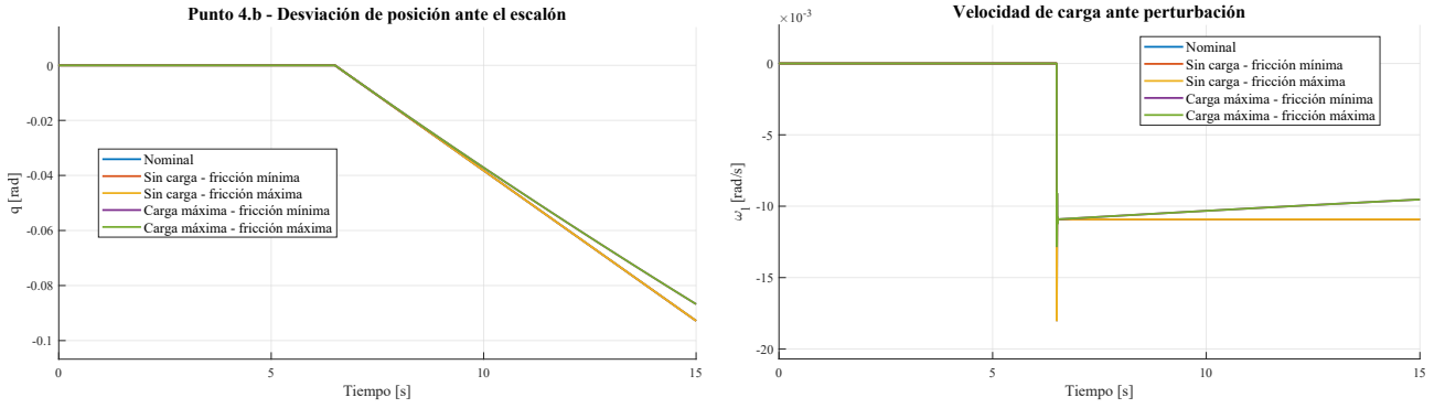
(a) Posición real de la carga para las distintas condiciones mecánicas. (b) Velocidad real de la carga ante el escalón de torque.
