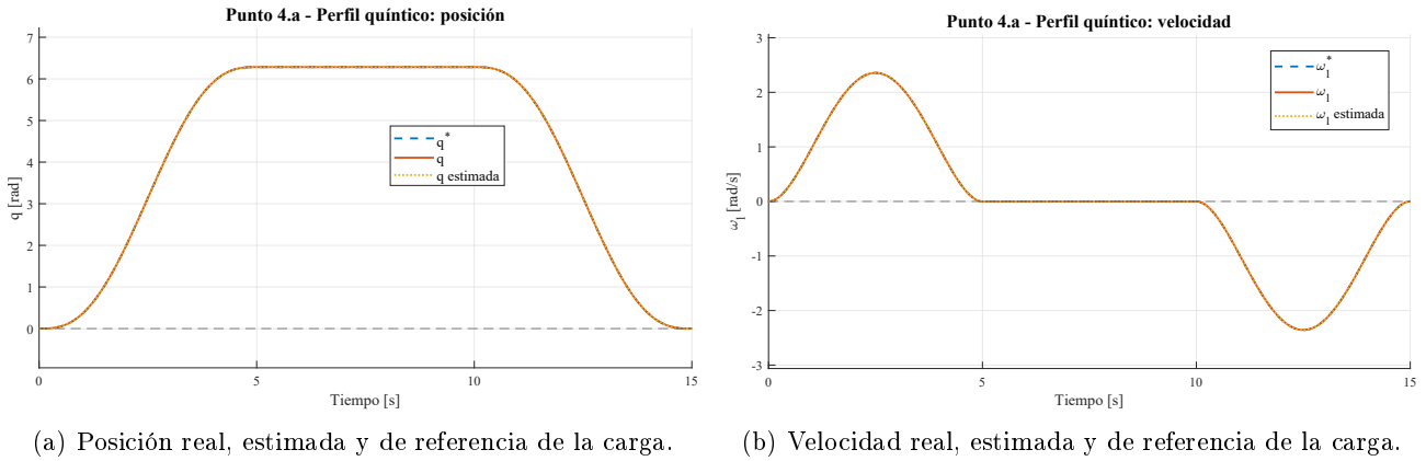
Figura 77: Seguimiento de posición y velocidad para el perfil polinómico de quinto orden.
