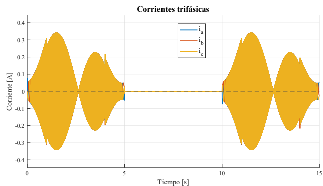
(b) Corrientes trifásicas del estator.
