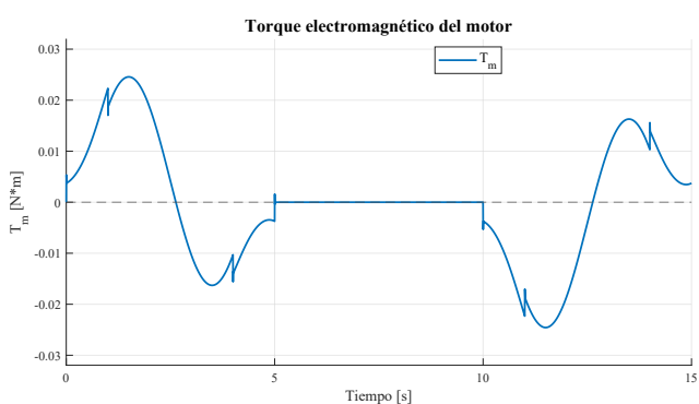
(a) Torque electromagnético desarrollado por el motor.
