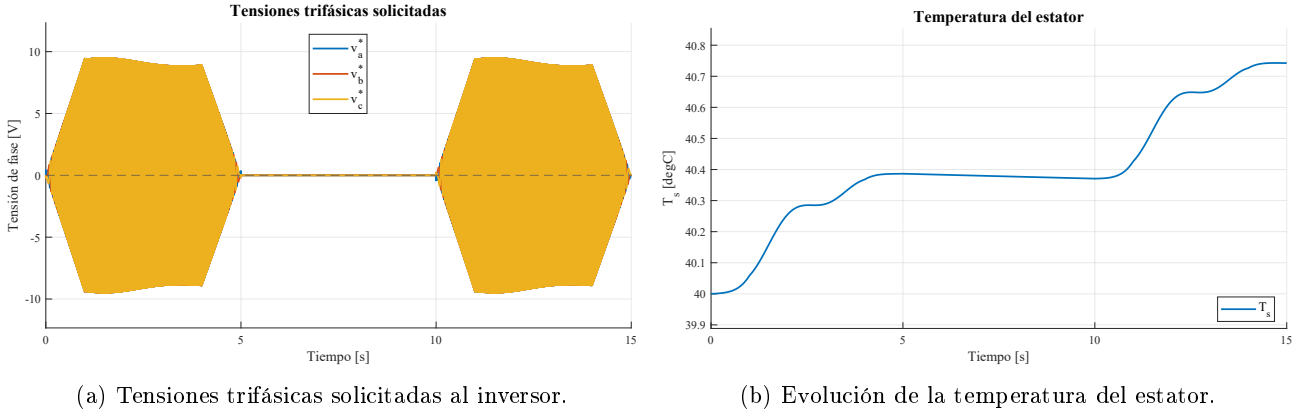
Figura 76: Tensiones solicitadas y respuesta térmica para la consigna trapezoidal de velocidad.
