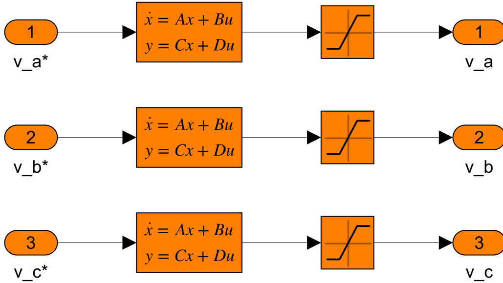
Figura 87: Diagrama de bloques del Modulador Trifásico de Tensión No Ideal en Simulink. A la izquierda se observa la estructura interna por fase incorporando la saturación estricta ( \pm 39,19 \text{ V} ) y la degradación dinámica en Espacio de Estados; a la derecha, el bloque consolidado.
