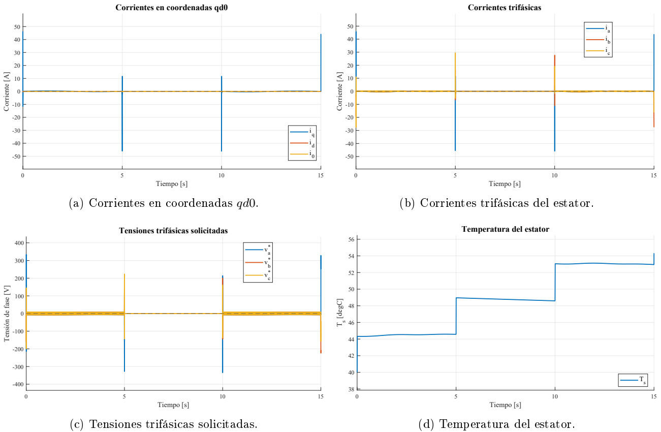
Figura 69: Corrientes, tensiones solicitadas y evolución de la temperatura del estator durante el seguimiento de la consigna.
