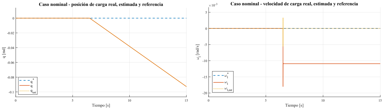
(a) Posición real, estimada y de referencia de la carga. (b) Velocidad real, estimada y de referencia de la carga.
