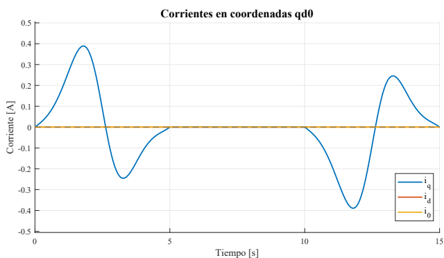
(a) Corrientes en coordenadas qd0 .
