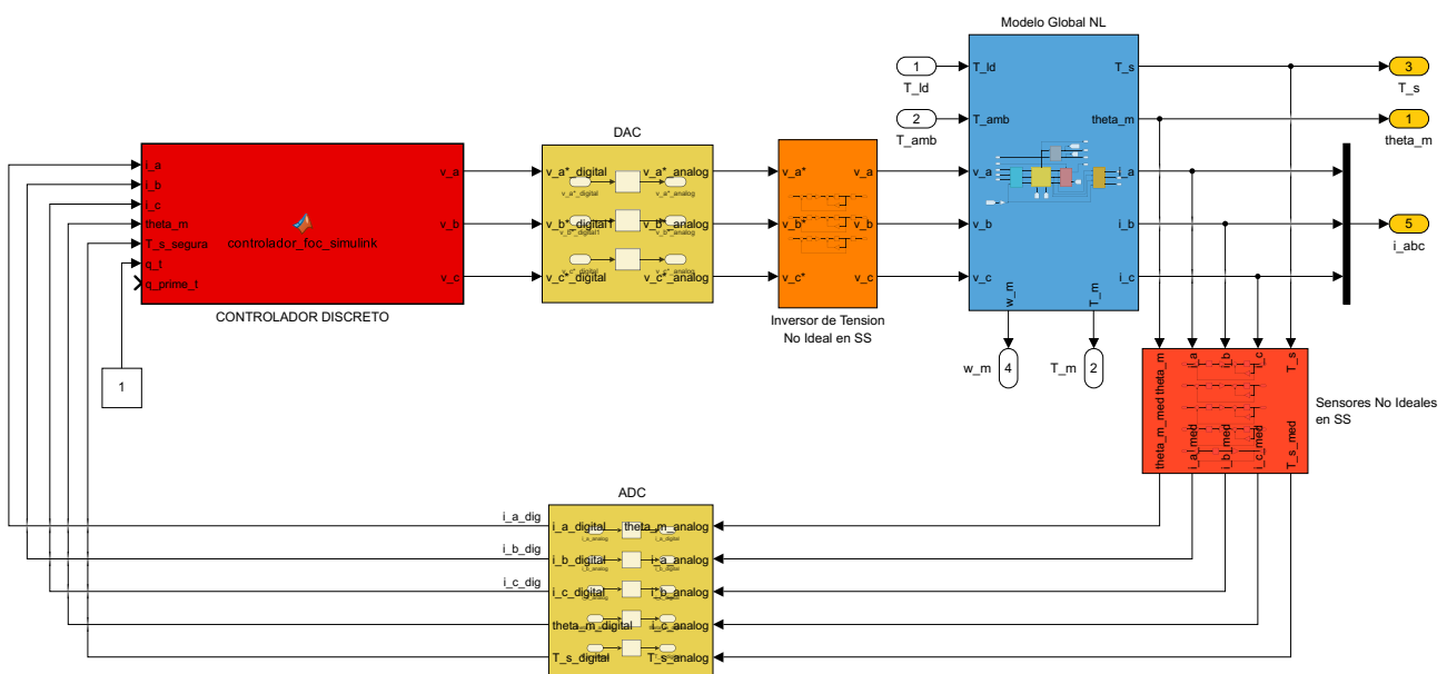
Figura 104: Arquitectura del controlador discreto programado mediante lenguaje de texto estructurado.
