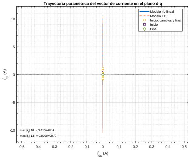
Figura 37: Trayectoria paramétrica del vector de corriente en el plano d-q .
