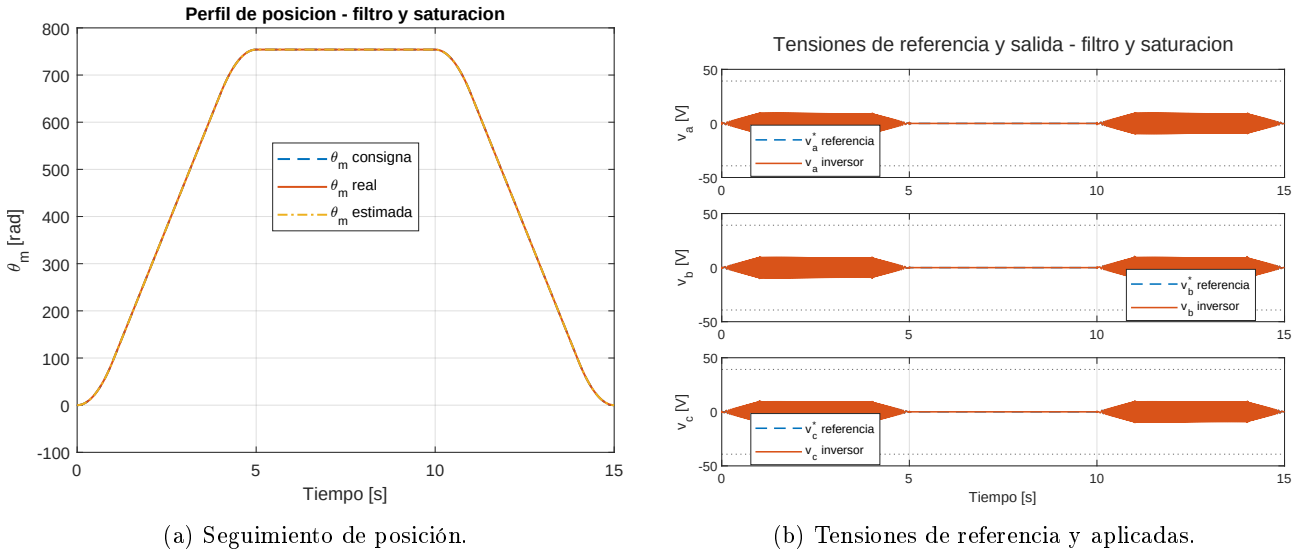
Figura 92: Respuesta del inversor completo para \omega_{n,v} = 27000 rad/s.
