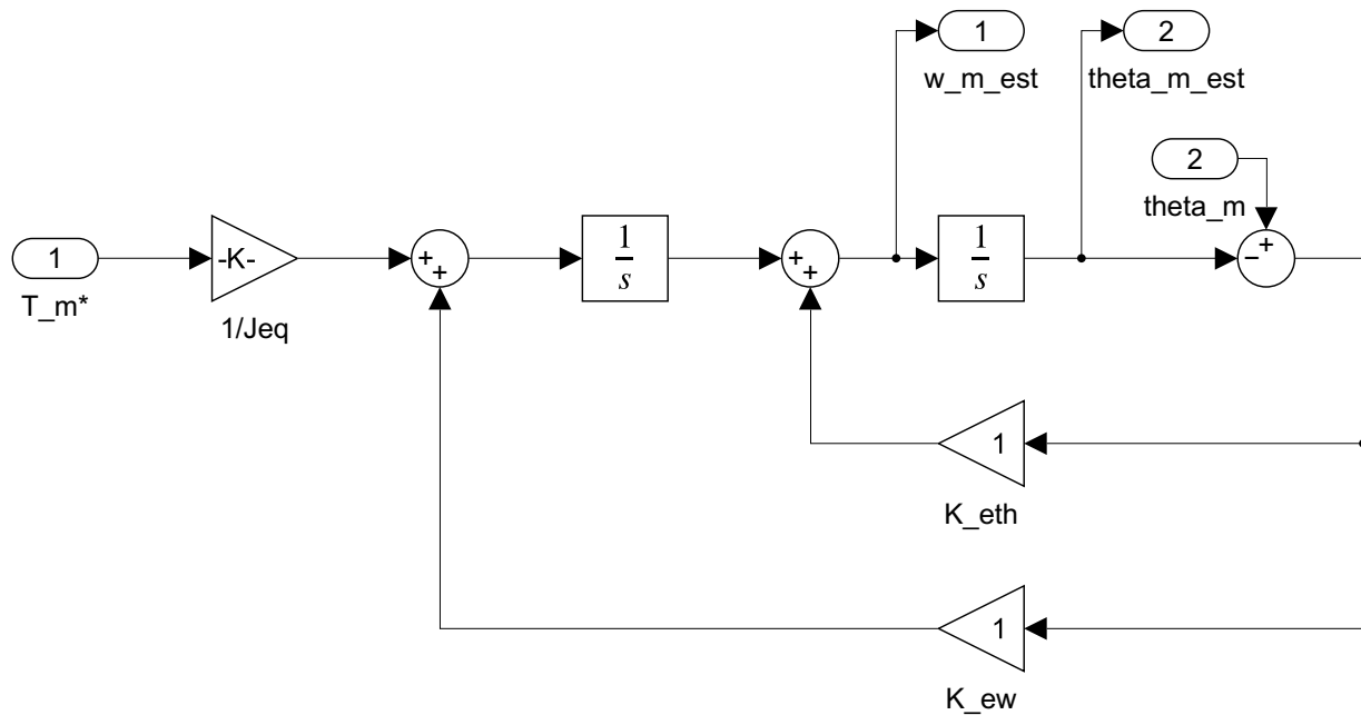
Figura 62: Diagrama de bloques del Observador de Estado Cinemático de orden reducido implementado en Simulink.
