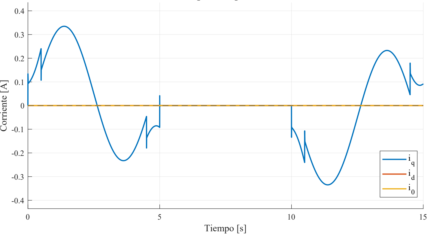
Corrientes qd0 con perfil suavizado
