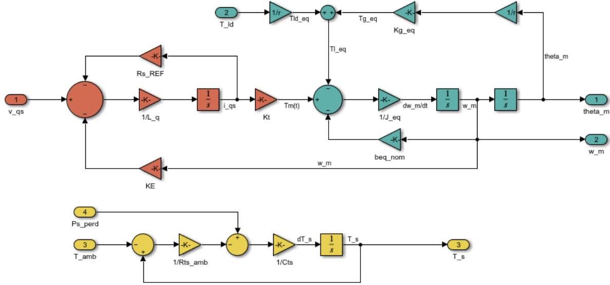
Figura 7: Diagrama de bloques del modelo LTI electromecánico equivalente por realimentación no lineal. Se muestra la dinámica principal de tres estados v_{qs}^r(t) \rightarrow i_{qs}^r(t) \rightarrow T_m(t) \rightarrow \omega_m(t) \rightarrow \theta_m(t) , junto con la perturbación mecánica externa, la gravedad linealizada y la rama térmica auxiliar excitada por P_{s,perd}(t) .
