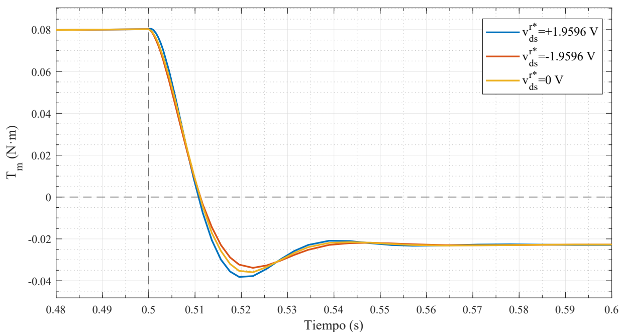
Figura 44: Torque electromagnético del modelo no lineal ante reforzamiento y debilitamiento de campo.
