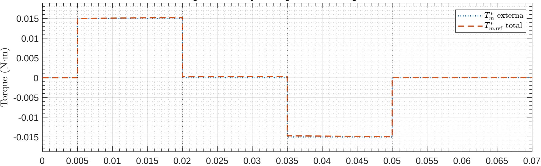
Aporte de compensación de fricción y gravedad
