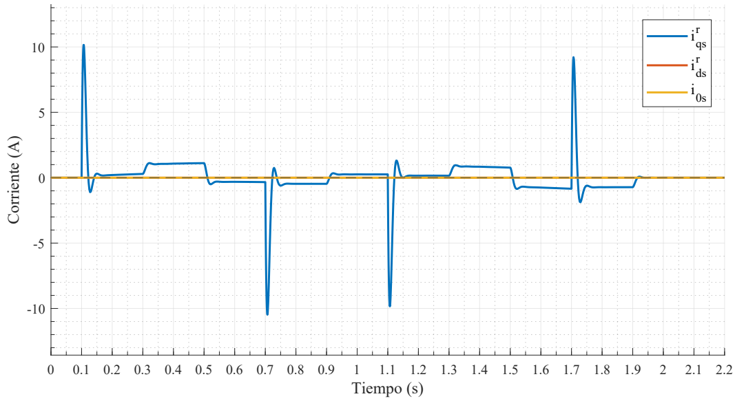
Figura 24: Corrientes estadísticas i_{qs}^r(t) , i_{ds}^r(t) e i_{0s}(t) , expresadas en coordenadas virtuales qd0 .
