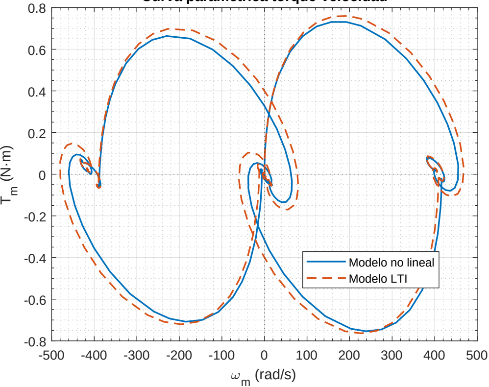
Curva paramétrica torque-velocidad
