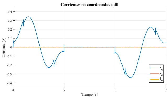
(a) Corrientes en coordenadas qd0 .
