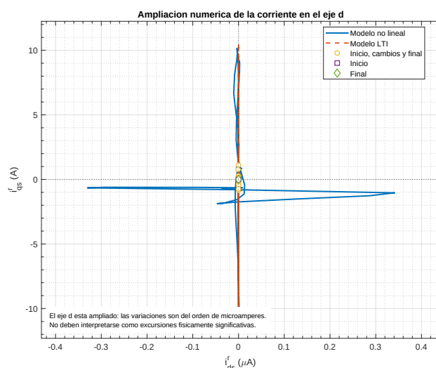
Figura 38: Ampliación de la trayectoria en el eje d , expresado en microamperes.
