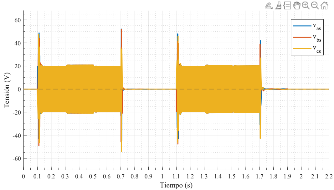
Figura 25: Tensiones estadóricas de fase v_a(t) , v_b(t) y v_c(t) , expresadas en coordenadas abc .
