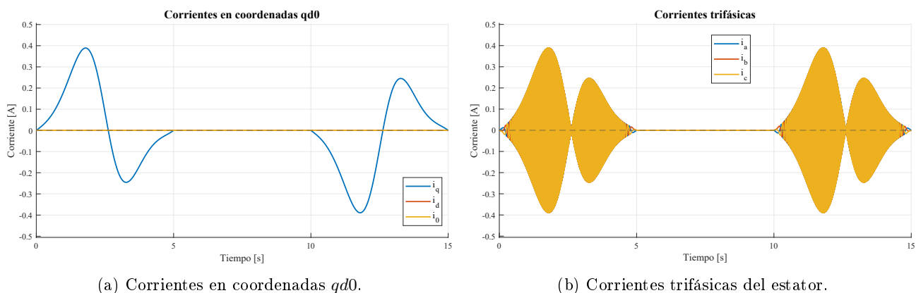
Figura 73: Corrientes del motor para el perfil polinómico de quinto orden.
