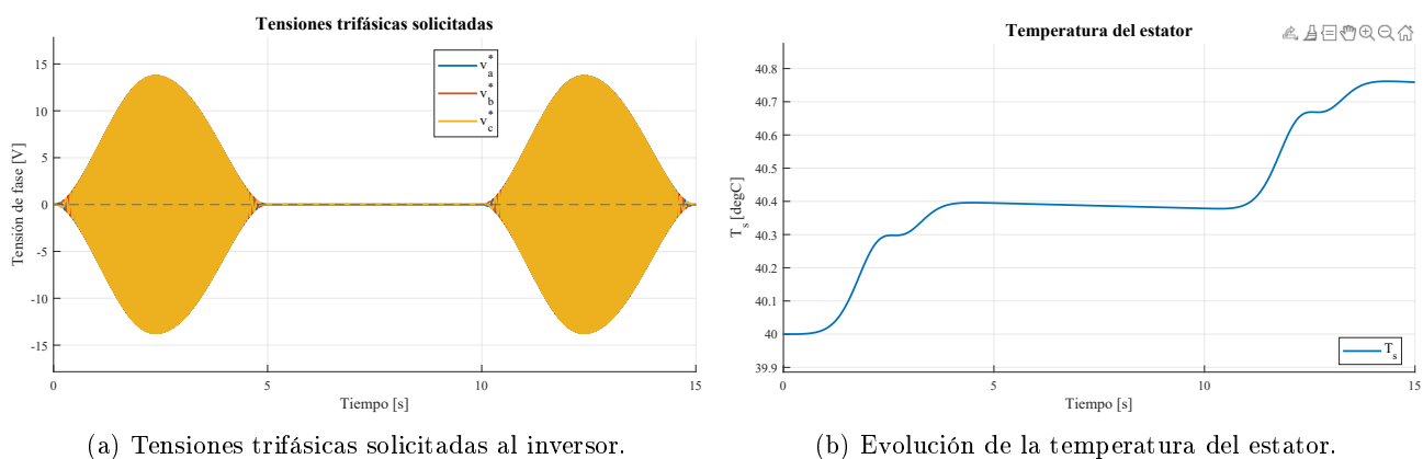
Figura 74: Tensiones solicitadas y respuesta térmica para el perfil polinómico de quinto orden.
