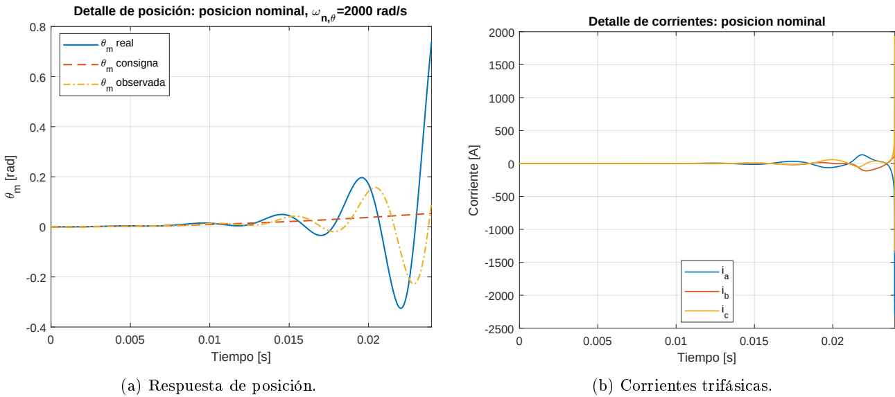
Figura 85: Respuesta del sistema con el sensor de posición nominal, \omega_{n,\theta} = 2000 \text{ rad/s} : (a) divergencia de la posición real y observada; (b) crecimiento no admisible de las corrientes de fase.
