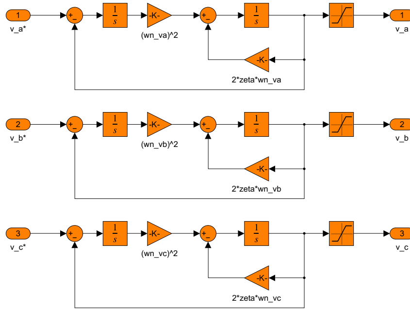
Figura 89: Diagrama de bloques del Modulador Trifásico de Tensión No Ideal en Simulink. Diagrama desagregado por fase incorporando la saturación estricta ( \pm 39,19 V) y la degradación dinámica en Espacio de Estados.
