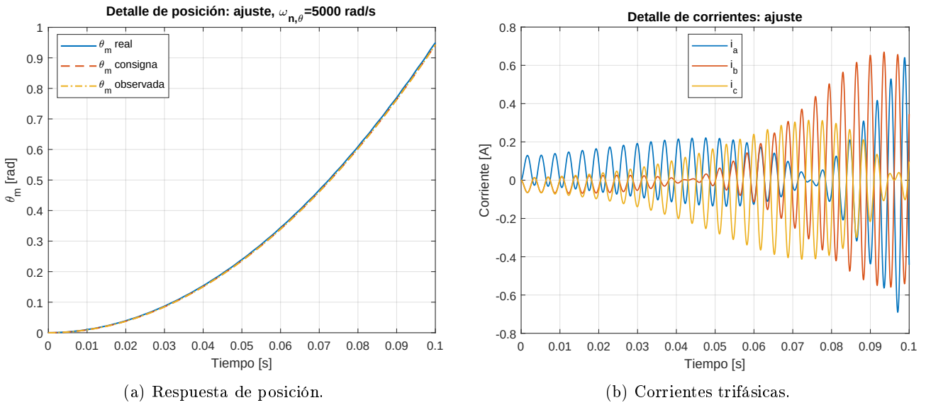
Figura 86: Respuesta del sistema con el sensor de posición ajustado a \omega_{n,\theta} = 5000 rad/s: (a) seguimiento adecuado de posición; (b) oscilaciones todavía presentes en las corrientes de fase.
