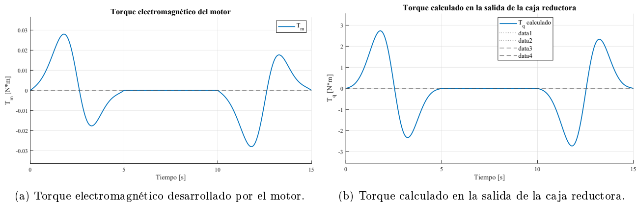
Figura 72: Torque electromagnético y torque de salida para el perfil polinómico de quinto orden.
