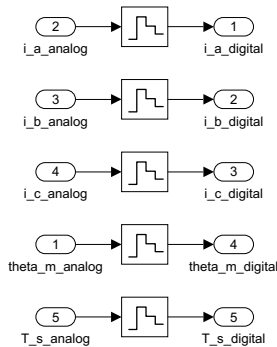
Figura 93: Conversores ADC implementados mediante retención de orden cero (ZOH).
