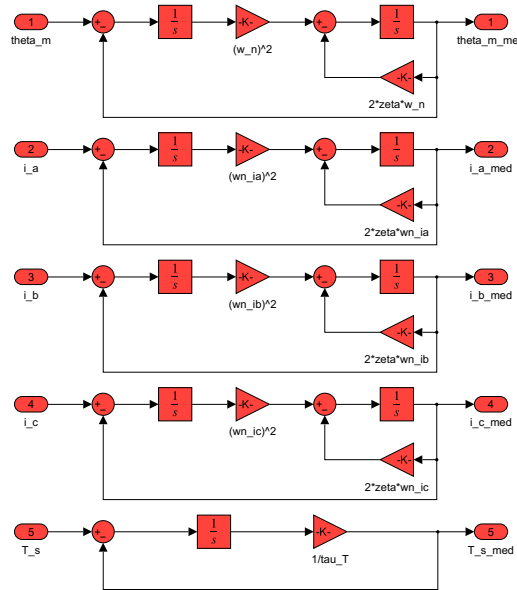
Figura 84: Diagrama de bloques implementado en Simulink para el modelo no ideal de sensores.
