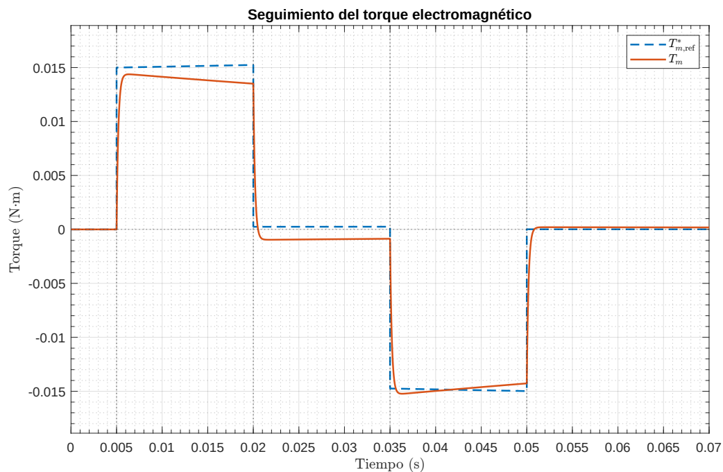
Figura 52: Seguimiento de la referencia electromagnética total por el torque generado por la máquina.
