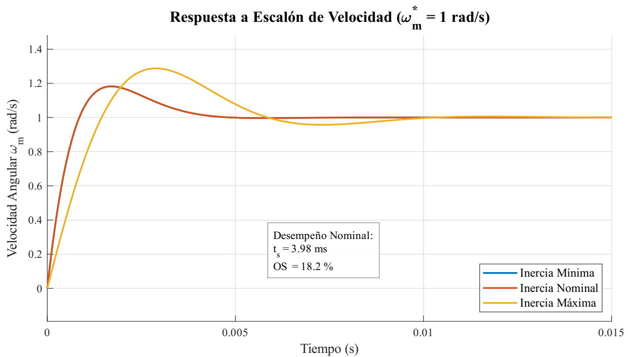
Figura 57: Respuesta del lazo de control frente a una entrada en escalón de velocidad.
