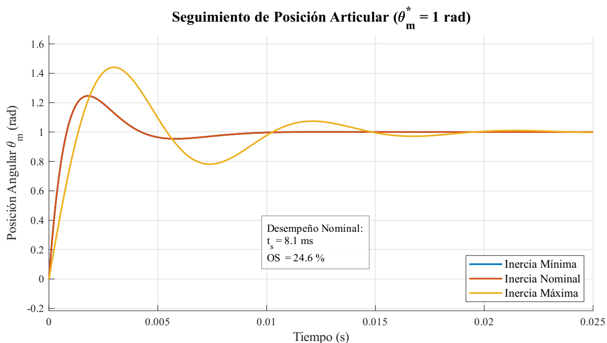
Figura 61: Respuesta del lazo de control frente a una entrada en escalón de posición.
