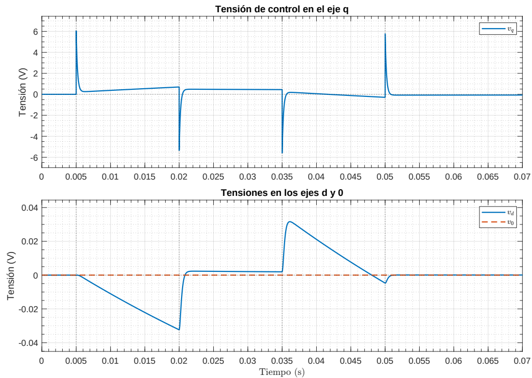
Figura 54: Tensiones de control generadas por el modulador en coordenadas qd0 .
