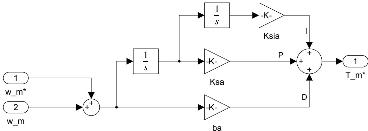
Figura 56: Implementación del controlador PID de movimiento en Simulink. La estructura utiliza integradores en cascada y una consigna de velocidad intermedia para evitar el uso de derivadores puros.
