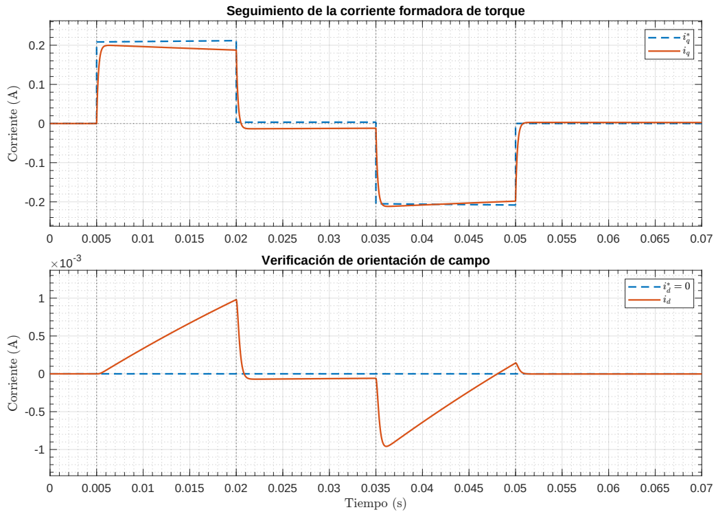
Figura 53: Seguimiento de las referencias de corriente en los ejes q y d .
