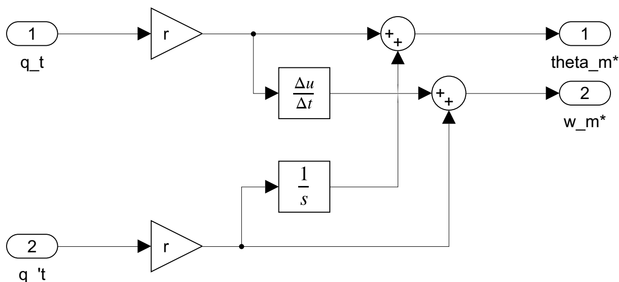
Figura 60: Implementación en Simulink de bloque set point.
