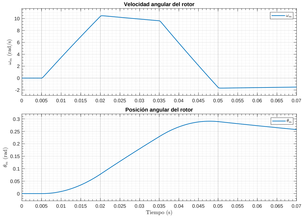
Figura 55: Respuesta mecánica producida por los pulsos de torque.
