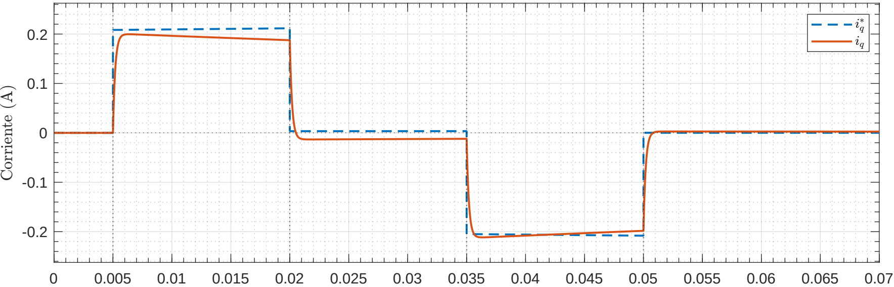
Seguimiento de la corriente formadora de torque
