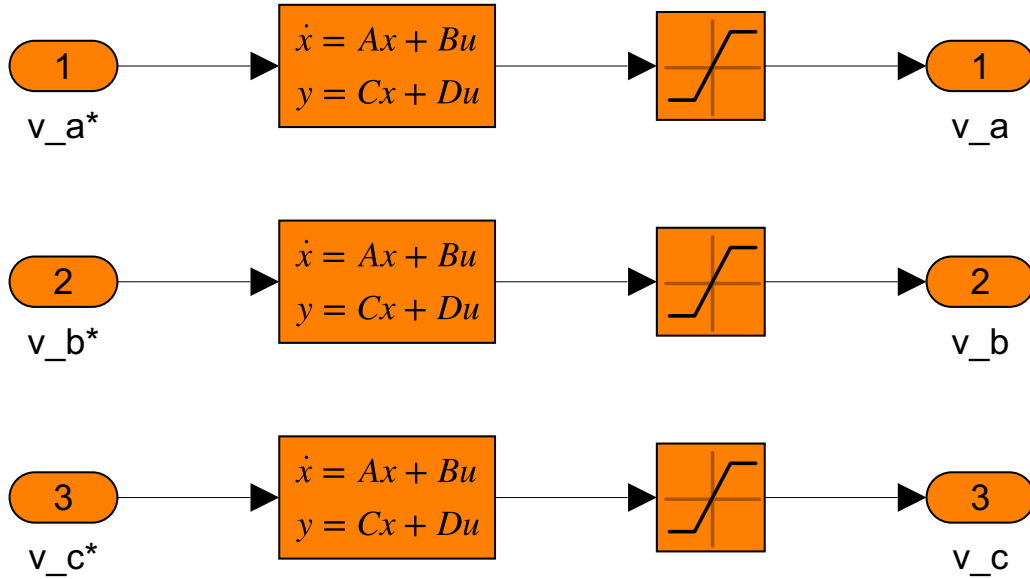
Figura 80: Diagrama de bloques del Modulador Trifásico de Tensión No Ideal en Simulink. A la izquierda se observa la estructura interna por fase incorporando la saturación estricta ( \pm 39,19 \text{ V} ) y la degradación dinámica en Espacio de Estados; a la derecha, el bloque consolidado.
