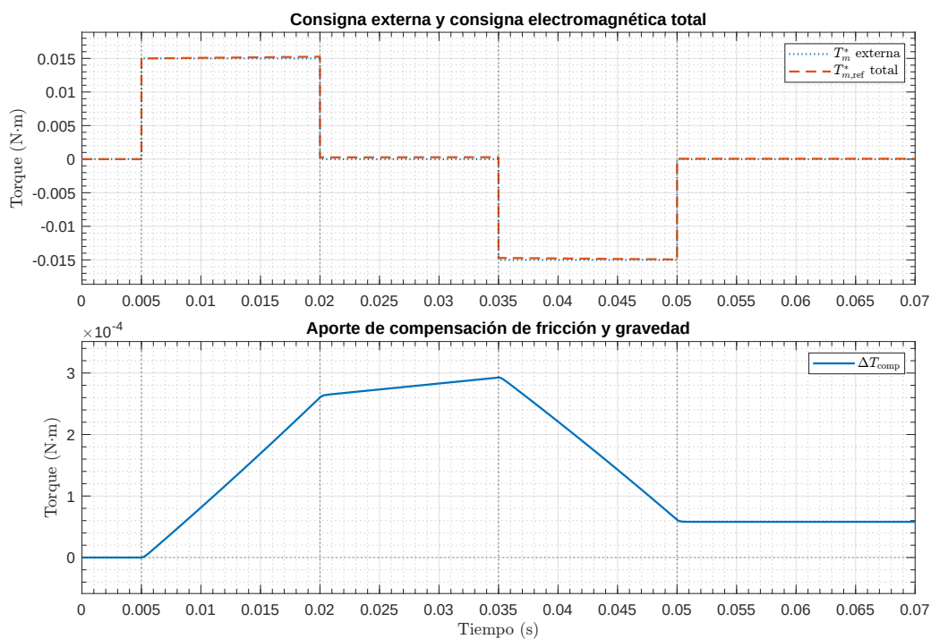
Figura 48: Consigna externa, referencia electromagnética total y aporte de la compensación de fricción y gravedad.
