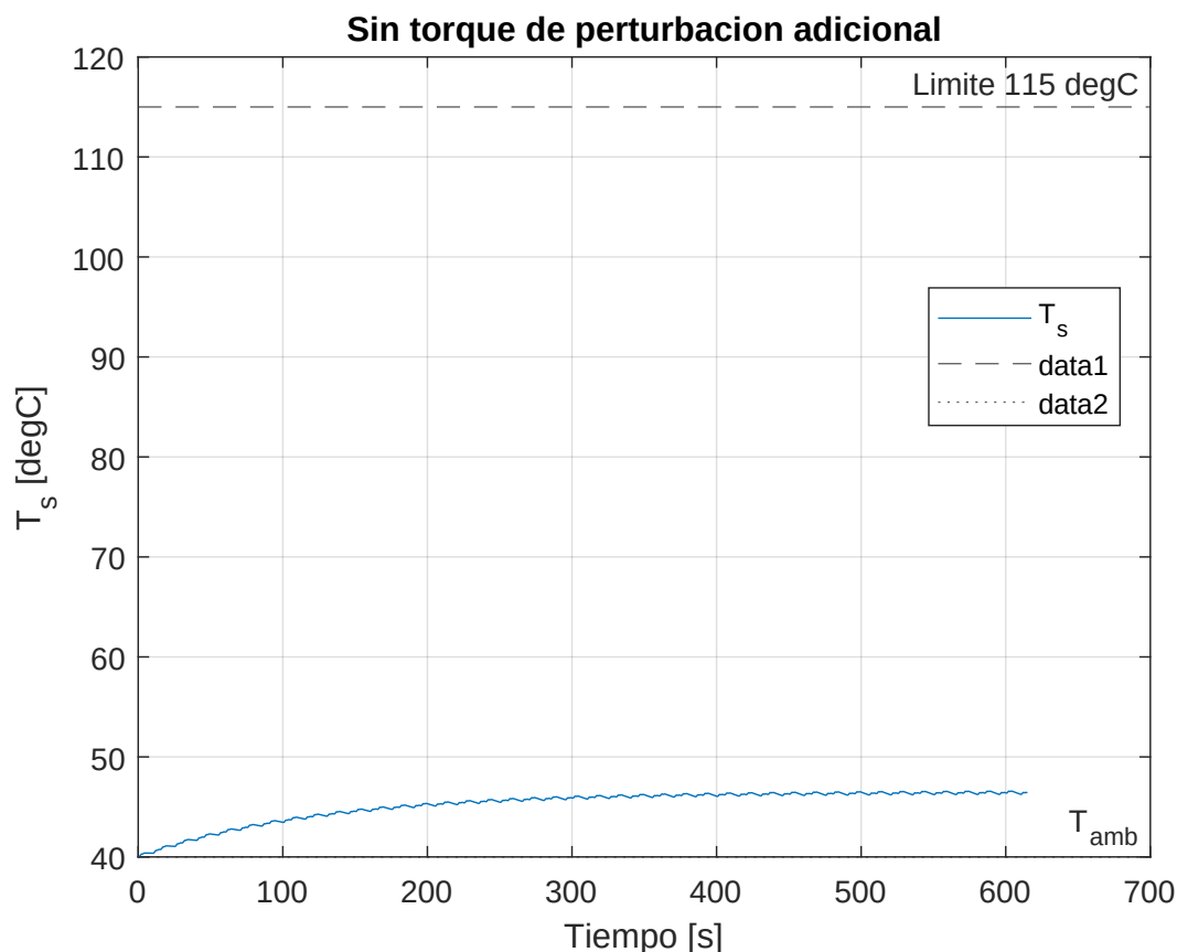
Figura 82: Temperatura del bobinado estático sin torque de perturbacion.
