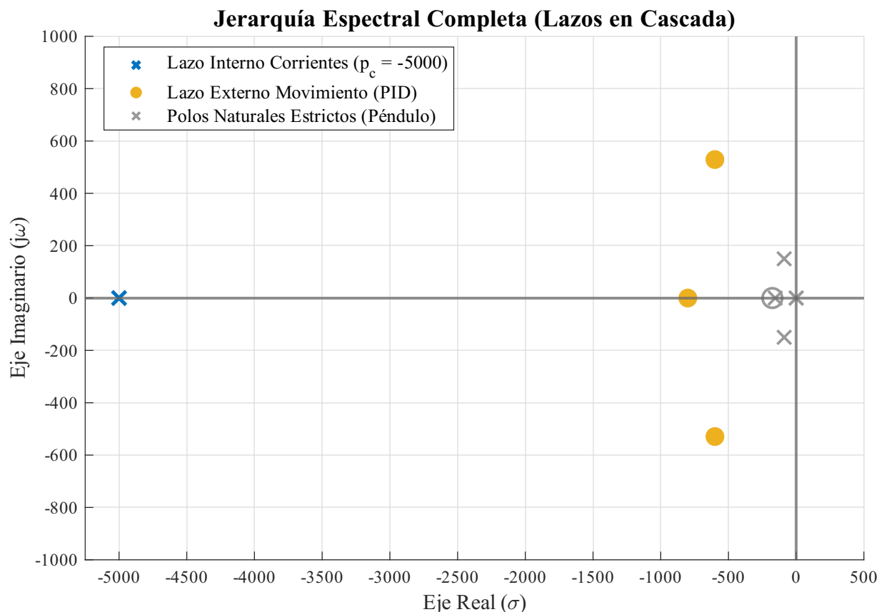
Figura 55: Jerarquía espectral de la arquitectura en cascada. Se observa la clara separación entre la dinámica dominante impuesta por el PID ( \omega_n = 800 ) y el lazo ultrarrápido de corriente ( p_c = -5000 ).
