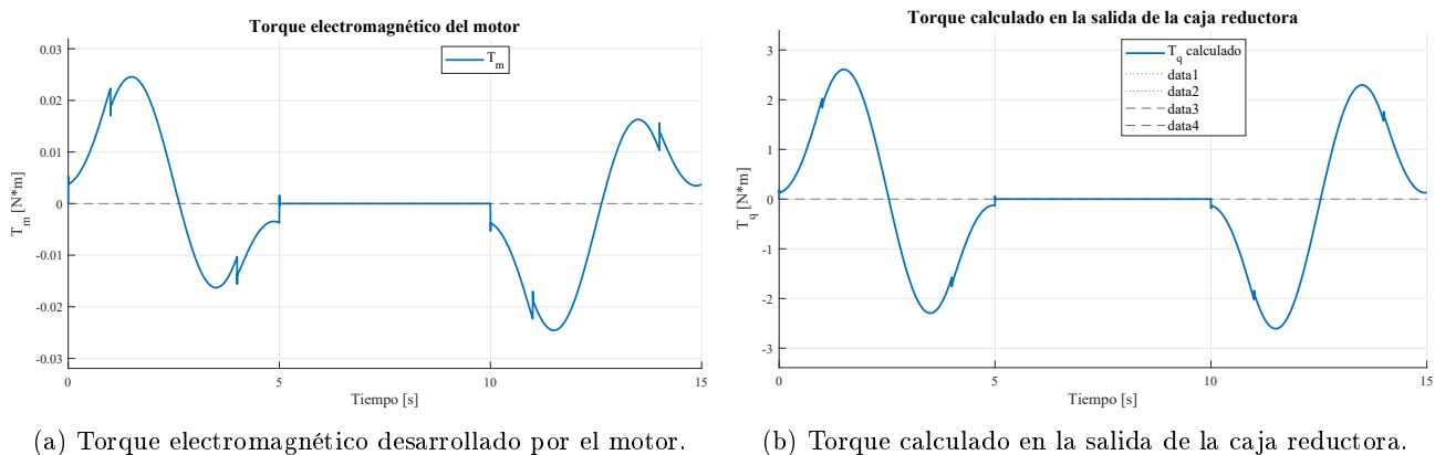
Figura 68: Torque electromagnético y torque de salida para la consigna trapezoidal de velocidad.
