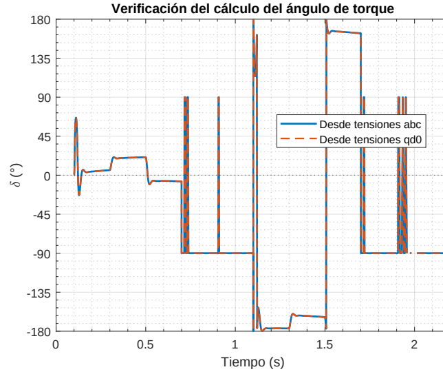
Figura 36: Verificación del cálculo de \delta(t) mediante las tensiones en coordenadas abc y qd0 .
