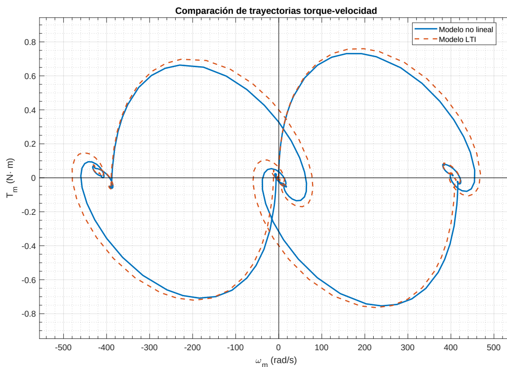
Figura 32: Comparación de las trayectorias paramétricas torque-velocidad obtenidas con el modelo no lineal y con el modelo LTI.
