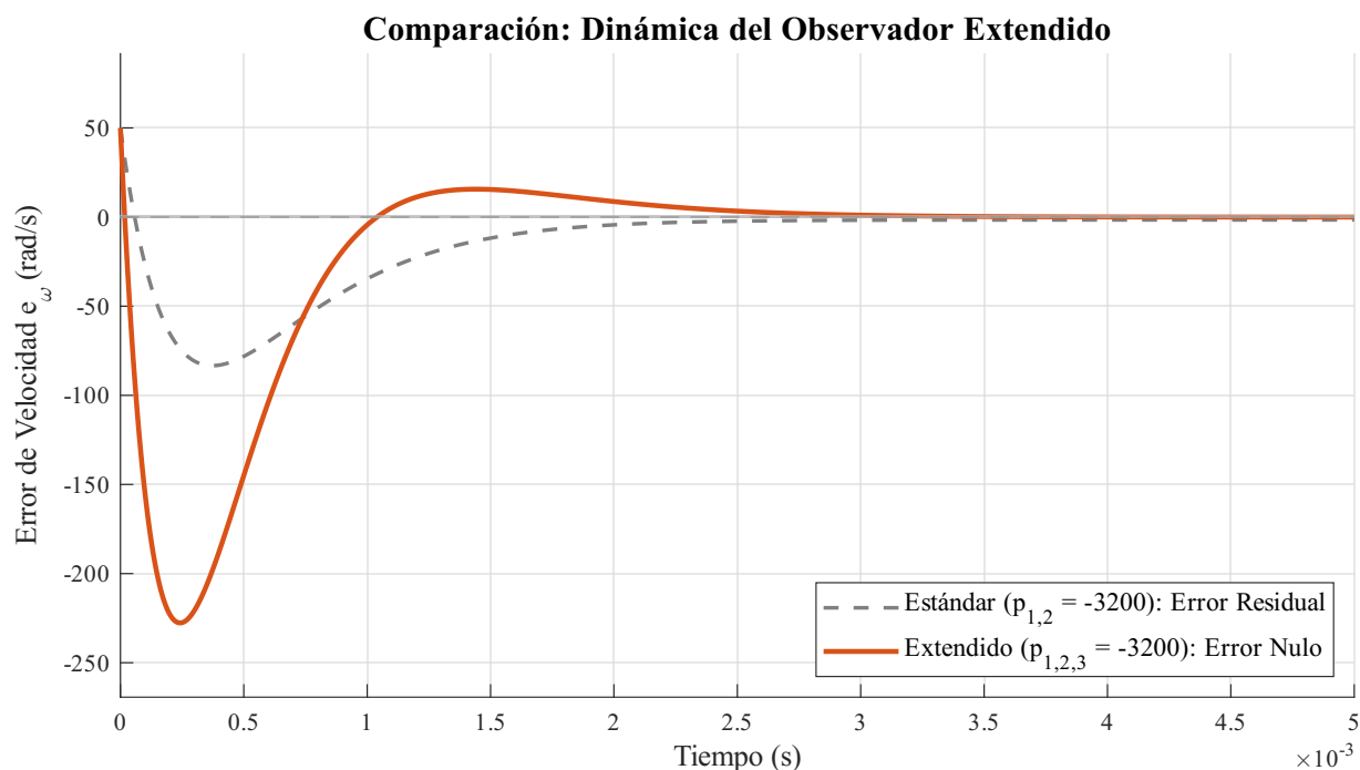
Figura 77: Efecto de la acción integral teórica. El observador extendido con polos en -3200 rad/s anula el error estacionario, pero induce un fenómeno de peaking perjudicial durante el transitorio inicial.
