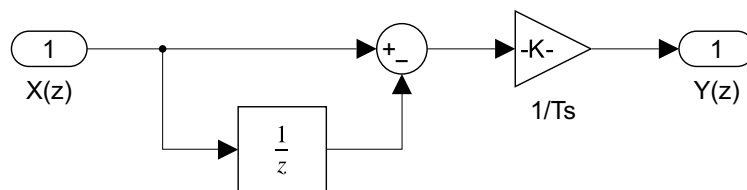
Figura 96: Estructura algorítmica desagregada para la derivación numérica mediante Diferencia Hacia Atrás.
