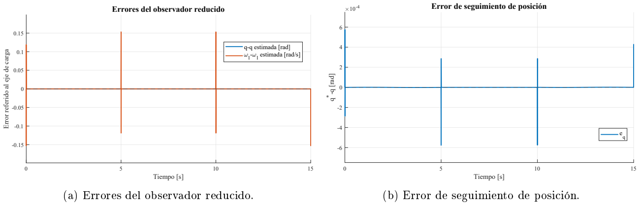
Figura 61: Errores de estimación y seguimiento obtenidos durante la simulación.
