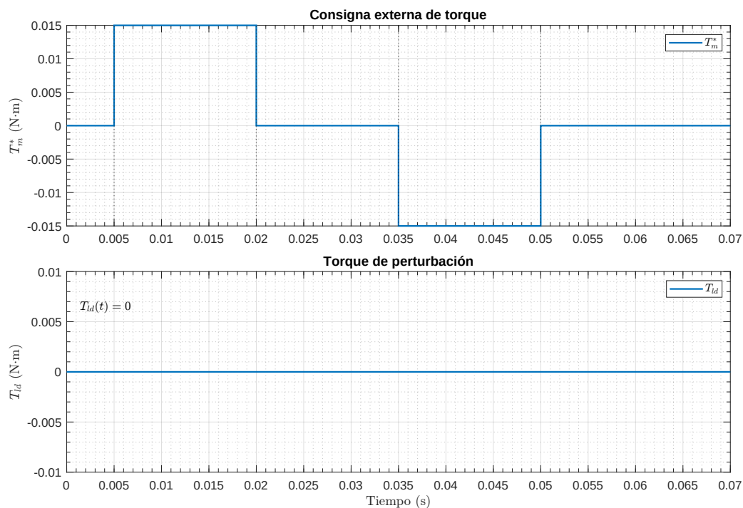
Figura 47: Consigna externa de torque y torque de perturbación utilizados en el ensayo del modulador.
