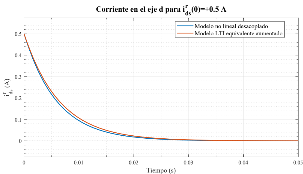
Figura 41: Evolución de i_{ds}^r(t) en los modelos no lineal desacoplado y LTI equivalente aumentado para i_{ds}^r(0) = +0,5 \text{ A} .
