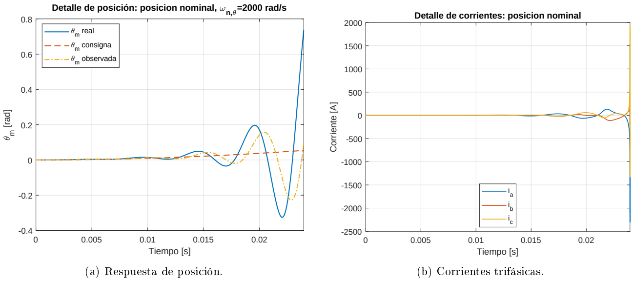
Figura 85: Respuesta del sistema con el sensor de posición nominal, \omega_{n,\theta} = 2000 rad/s: (a) divergencia de la posición real y observada; (b) crecimiento no admisible de las corrientes de fase.
