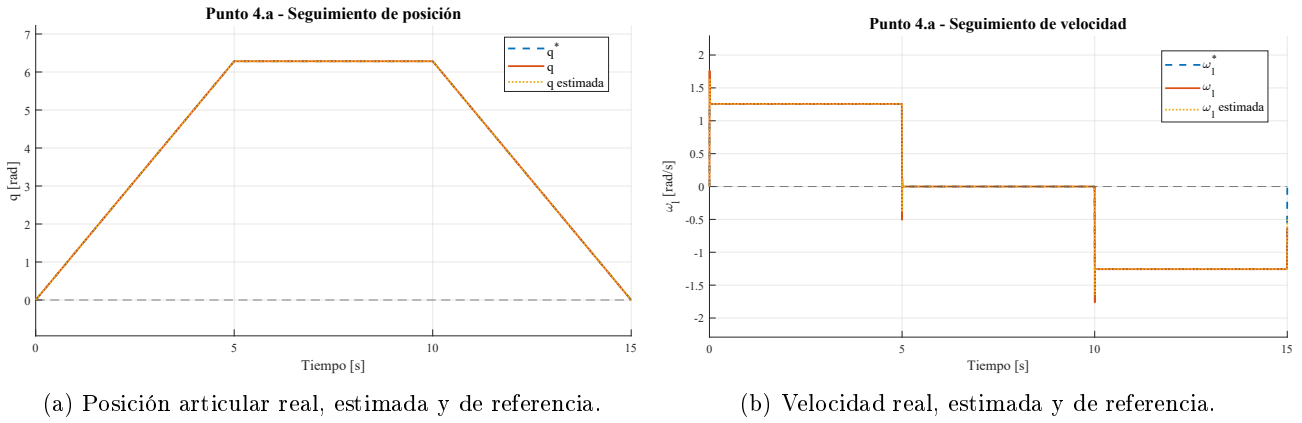
Figura 60: Seguimiento de la consigna de movimiento.
