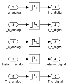
Figura 93: Conversores ADC implementados mediante retención de orden cero (ZOH).
