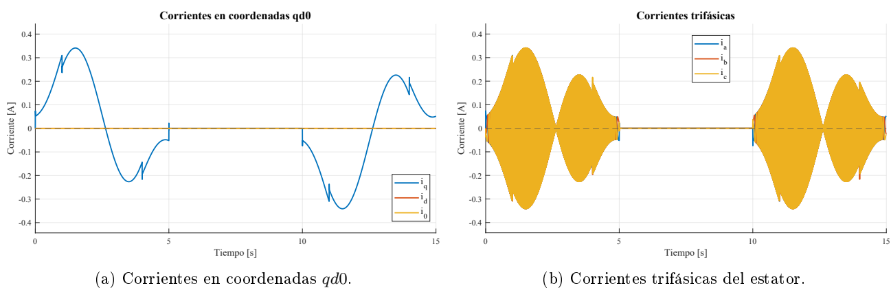
Figura 69: Corrientes del motor para la consigna trapezoidal de velocidad.
