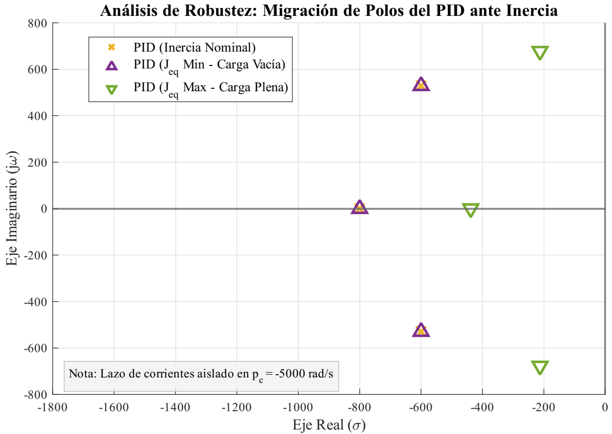
Figura 56: Migración de los polos dominantes del lazo PID ante variaciones de la inercia equivalente de carga ( J_{eq} ). La estabilidad asintótica se conserva en todos los escenarios.
