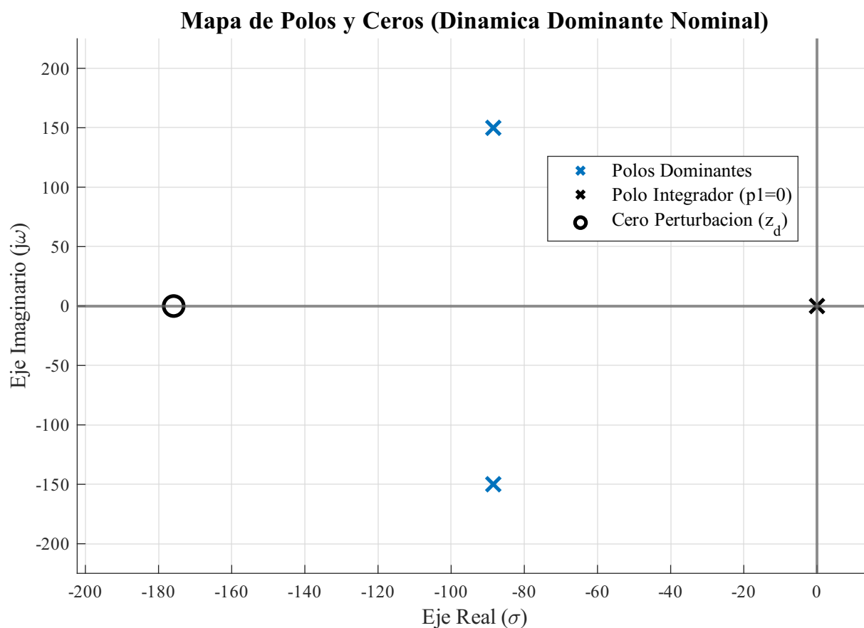
Figura 11: Mapa de polos y ceros nominal del modelo LTI equivalente.
