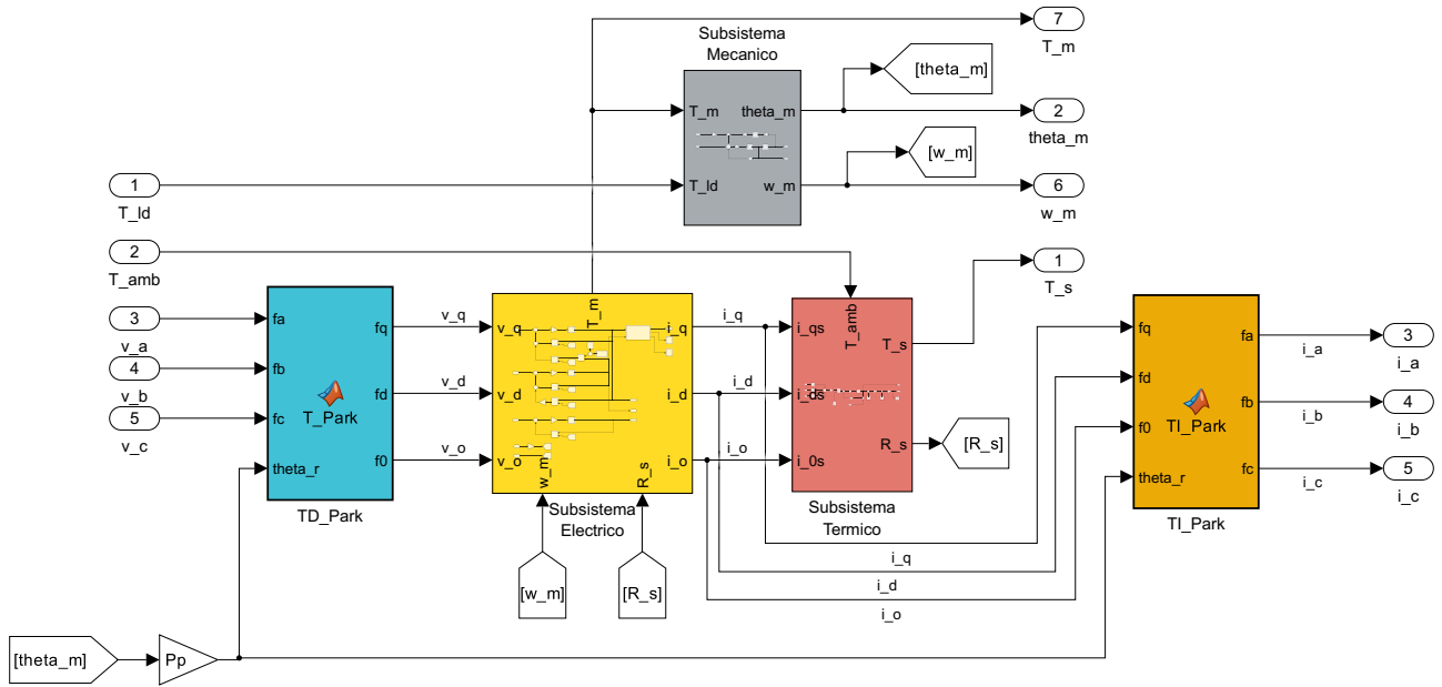
Figura 6: Modelo global no lineal del accionamiento PMSM implementado en Simulink. El diagrama integra las transformaciones de Park directa e inversa, el subsistema eléctrico en coordenadas qd0 , el subsistema mecánico equivalente, el cálculo térmico de pérdidas Joule y la retroalimentación de la resistencia estatórica variable R_s(T_s^\circ) .
