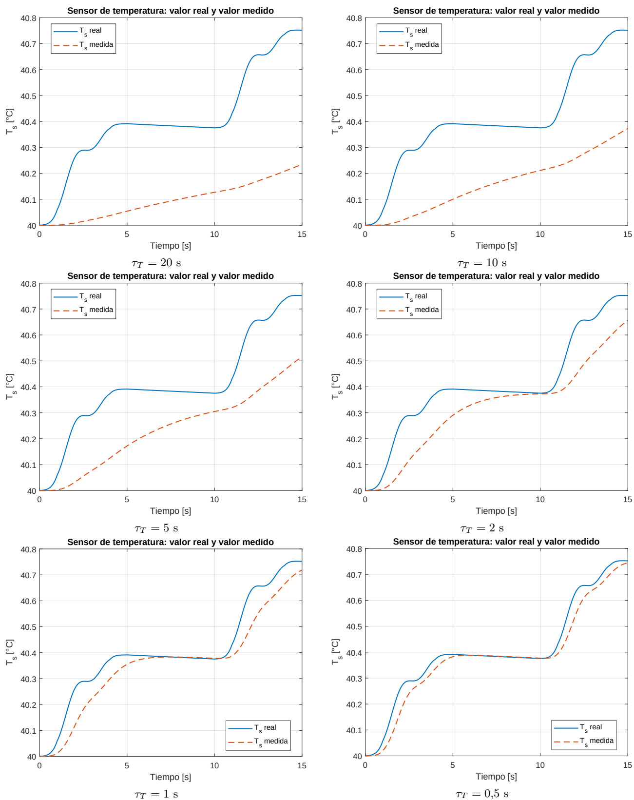
Figura 88: Comparación entre temperatura real y medida para diferentes constantes de tiempo del sensor térmico.
