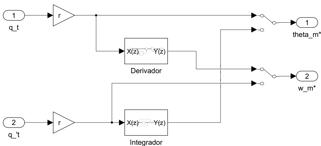
Figura 99: Implementación en tiempo discreto de la Interfaz de Referencia (Set-Point).
