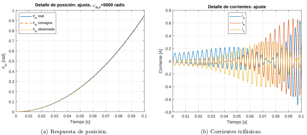
Figura 86: Respuesta del sistema con el sensor de posición ajustado a \omega_{n,\theta} = 5000 rad/s: (a) seguimiento adecuado de posición; (b) oscilaciones todavía presentes en las corrientes de fase.
