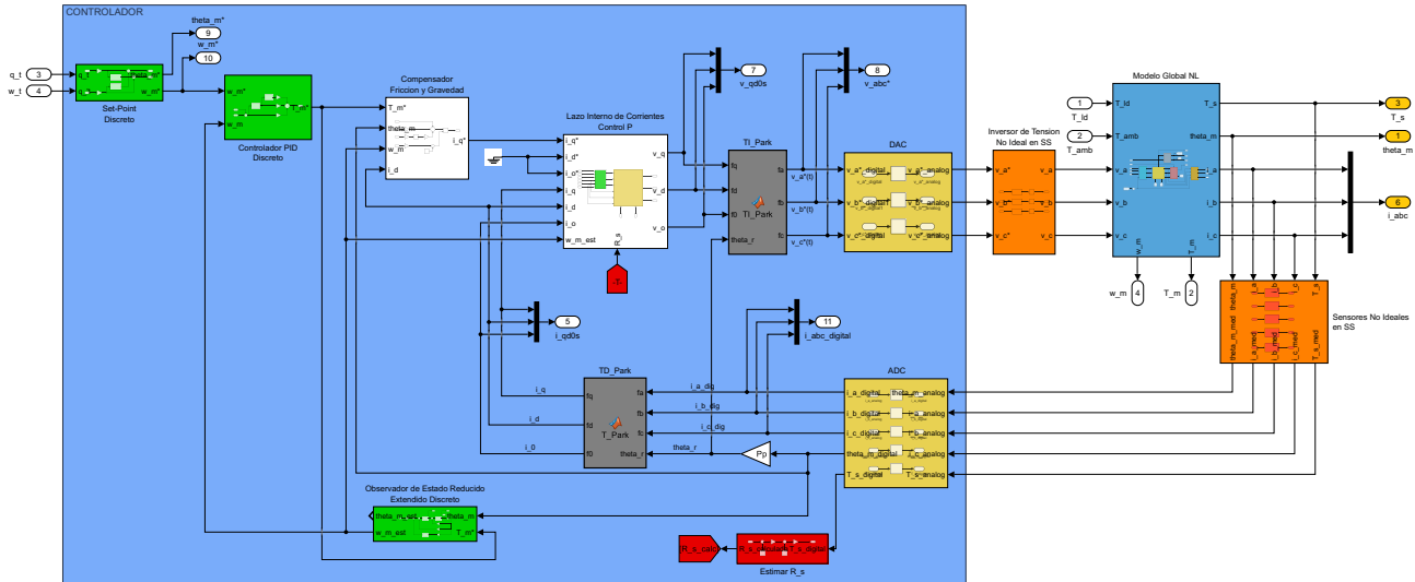
Figura 100: Arquitectura integral del controlador en cascada discretizado.
