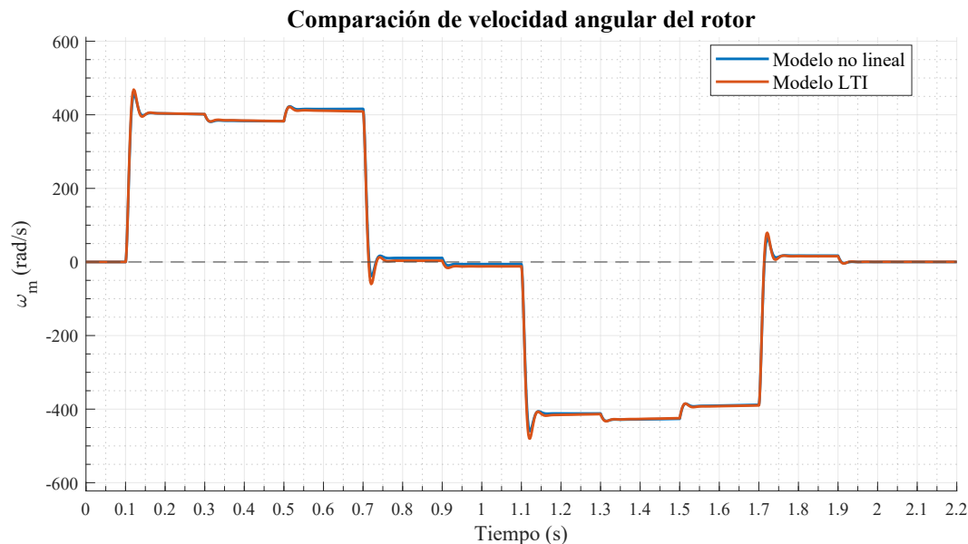
Figura 29: Comparación de la velocidad angular del rotor \omega_m(t) obtenida con los modelos no lineal y LTI.
