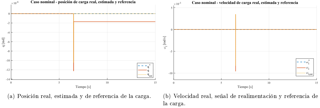
Figura 65: Respuesta del eje para caso nominal.
