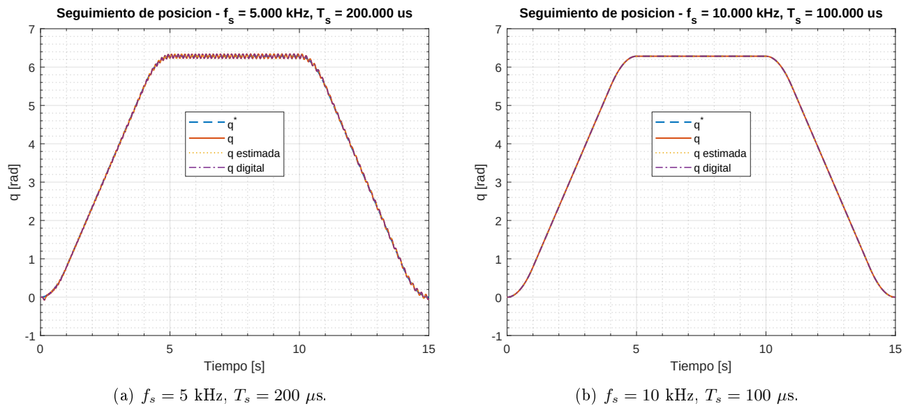
Figura 102: Detalle del efecto de la frecuencia de muestreo sobre la respuesta en posición.
