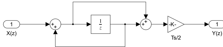
Figura 95: Implementación en bloques discretos elementales de la integración por el método de Tustin.
