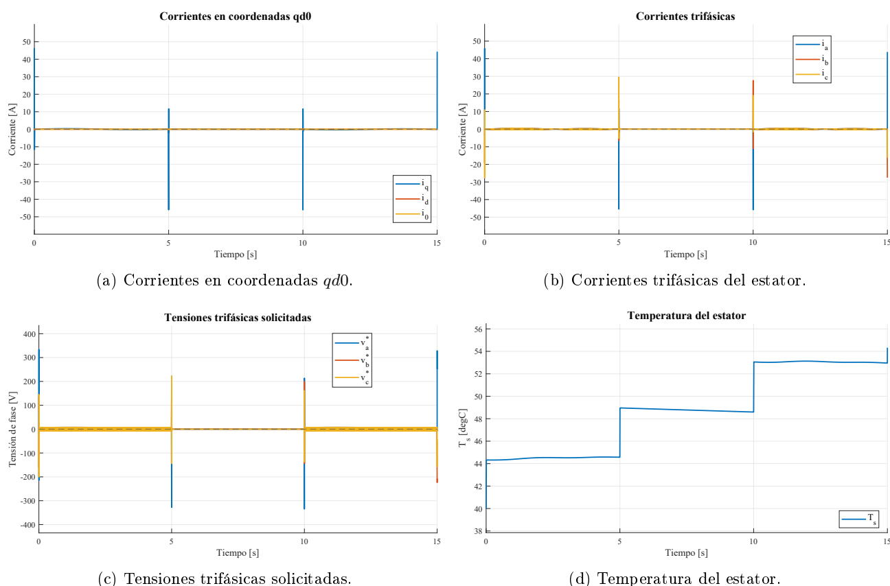
Figura 63: Corrientes, tensiones solicitadas y evolución de la temperatura del estator durante el seguimiento de la consigna.
