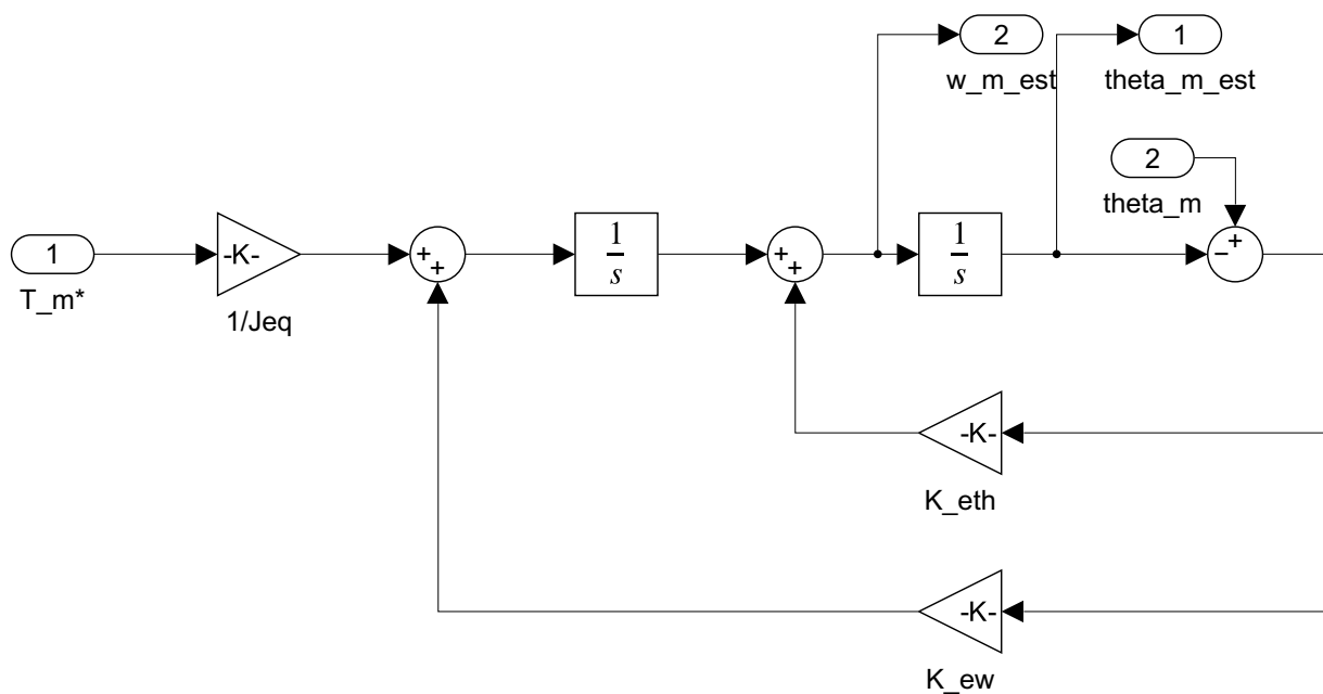
Figura 58: Diagrama de bloques del Observador de Estado Cinemático de orden reducido implementado en Simulink.
