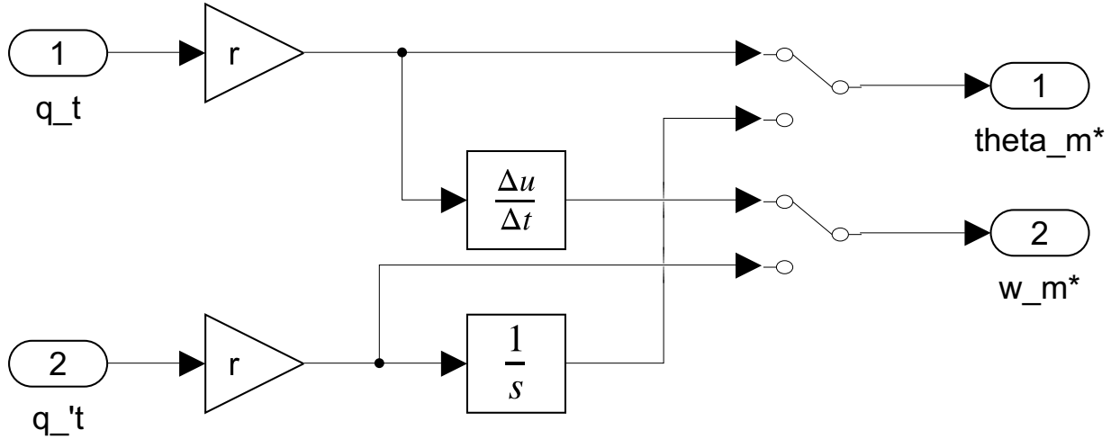
Figura 57: Implementación en Simulink de bloque set point.
