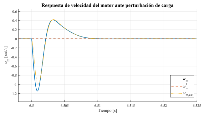
(b) Detalle de la velocidad real y de la derivada de la posición estimada.
