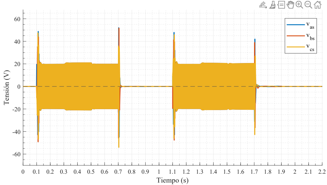
Figura 25: Tensiones estatóricas de fase v_a(t) , v_b(t) y v_c(t) , expresadas en coordenadas abc .
