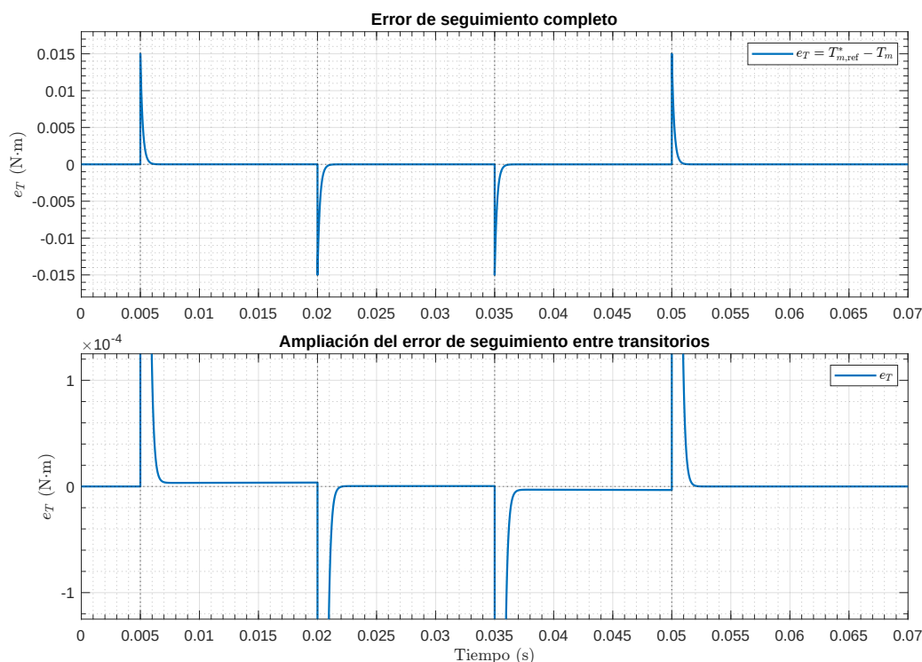
Figura 50: Error de seguimiento de torque completo y ampliación del comportamiento cuasiestacionario.
