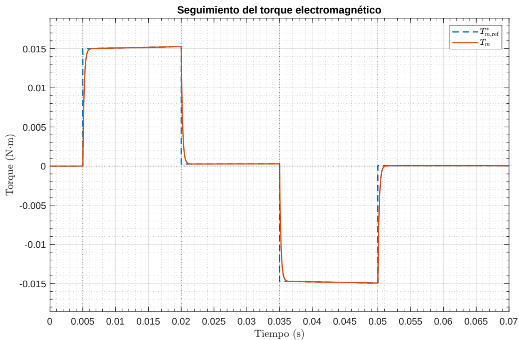
Figura 49: Seguimiento de la referencia electromagnética total por el torque generado por la máquina.
