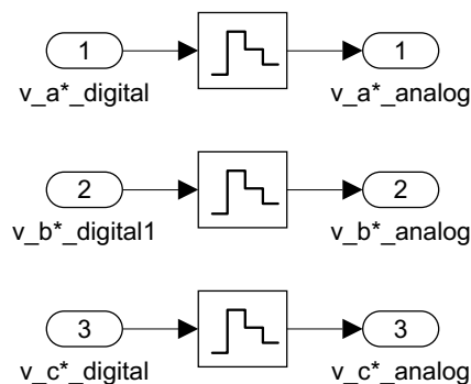
Figura 94: Conversores DAC implementados mediante retención de orden cero (ZOH), emulando un PWM.
