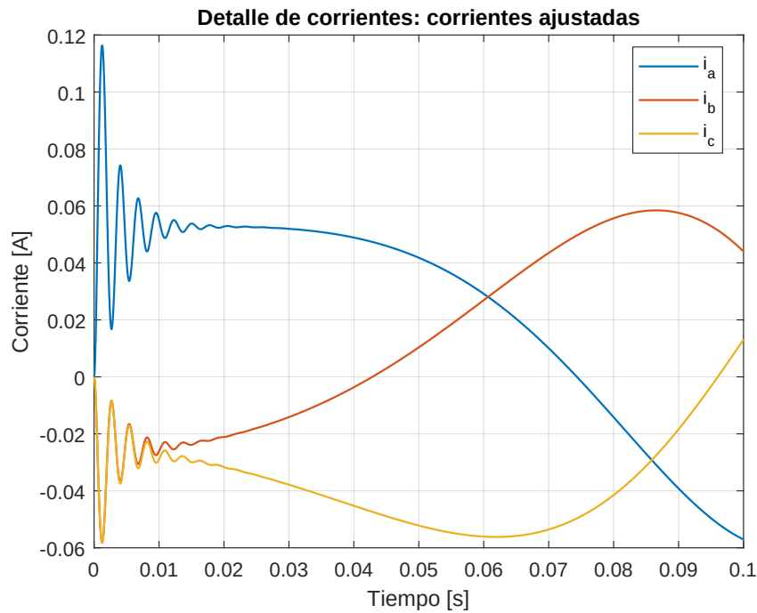
Figura 87: Corrientes trifásicas con \omega_{n,i} = 10000 rad/s.
