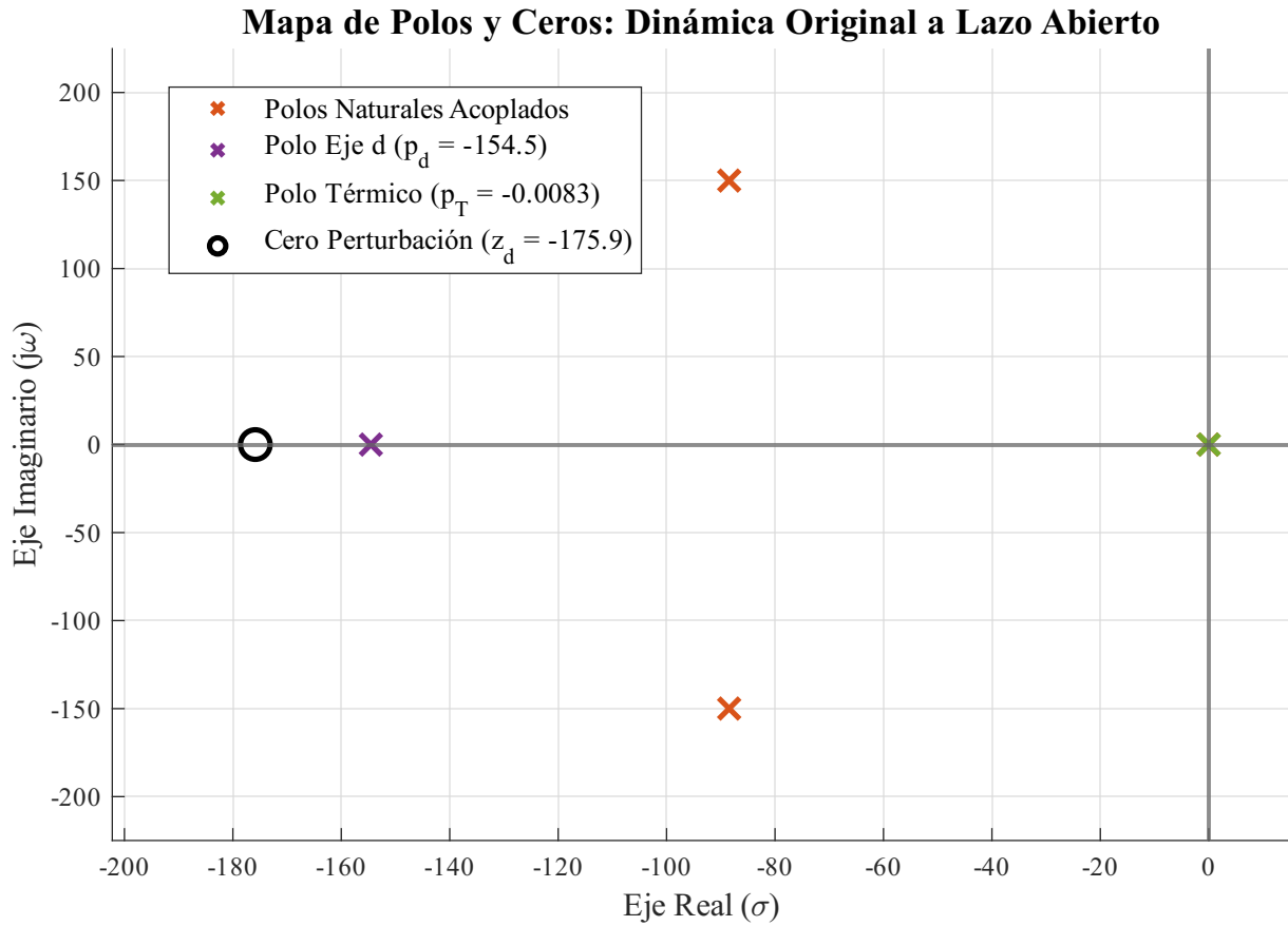
Figura 45: Mapa de polos y ceros del sistema no lineal original a lazo abierto. Constituye el punto de partida previo al diseño de las estrategias de desacoplamiento y control en cascada.
