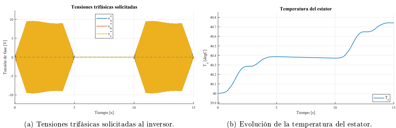
Figura 70: Tensiones solicitadas y respuesta térmica para la consigna trapezoidal de velocidad.
