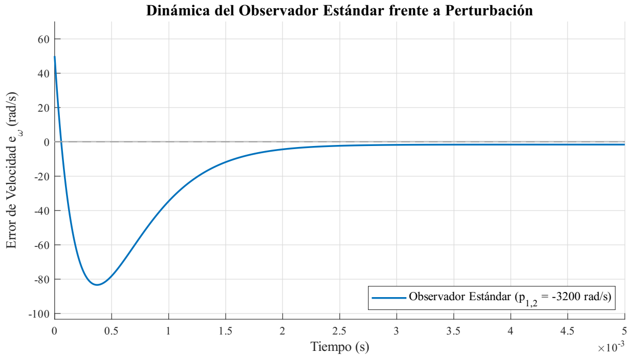
Figura 75: Dinámica del error de estimación del observador estándar de orden 2. Ante una perturbación de torque activa, el sistema presenta un error de velocidad residual.
