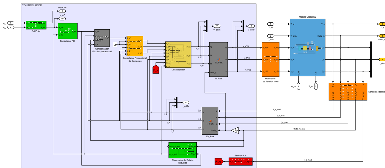
Figura 59: Diagrama Sistema de Control completo.
