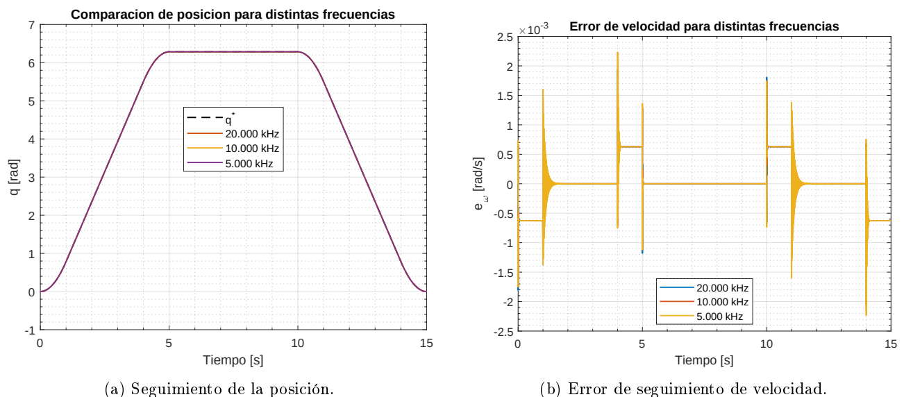
Figura 101: Comparación del desempeño para distintas frecuencias de muestreo.
