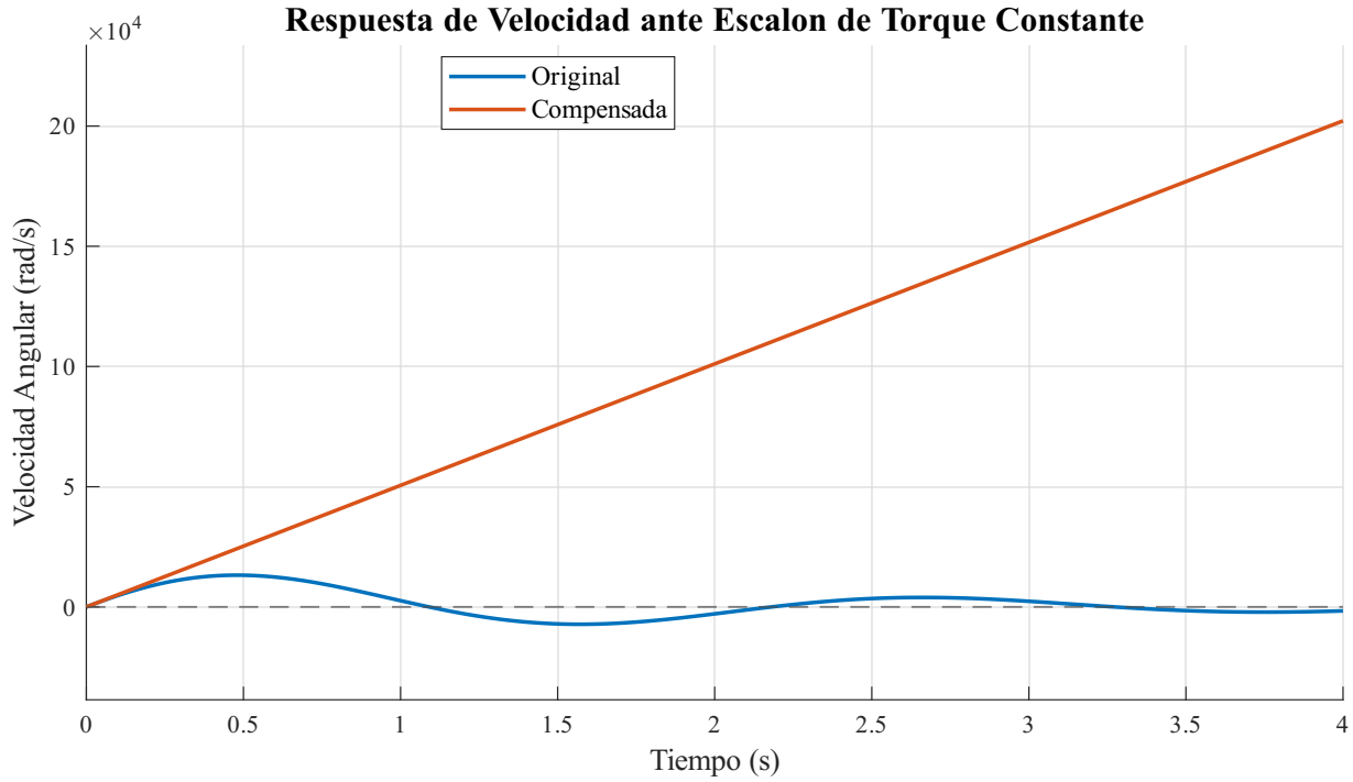
Figura 46: Comparativa de la respuesta de velocidad ante un escalón de torque: el sistema natural oscila hasta detenerse contrarrestando la gravedad, mientras que el sistema compensado responde como una inercia ideal (rampa de velocidad continua).
