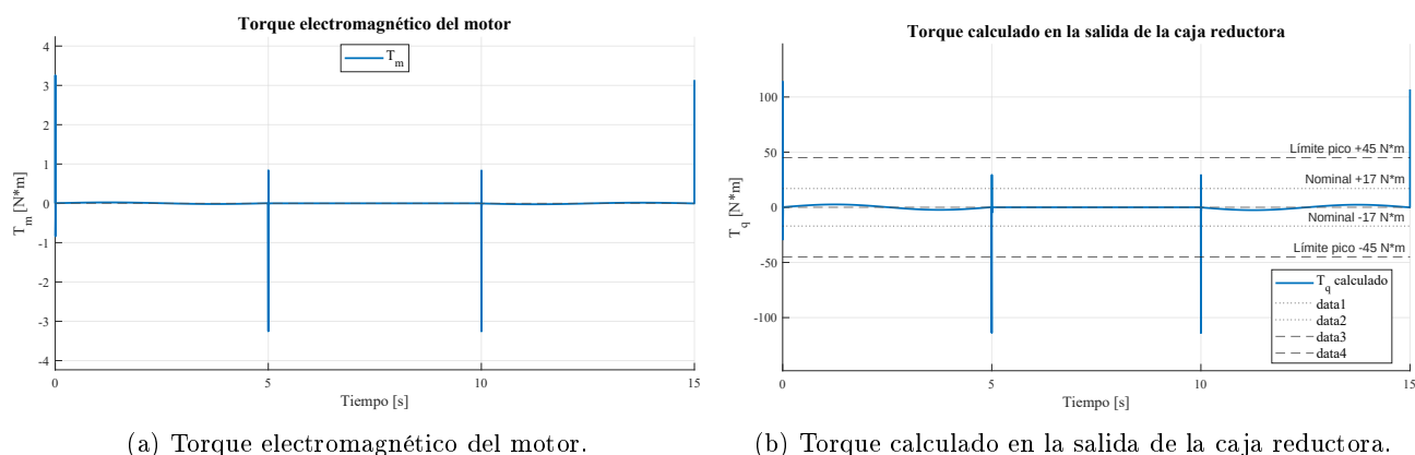
Figura 62: Torques requeridos para cumplir la consigna de movimiento.
