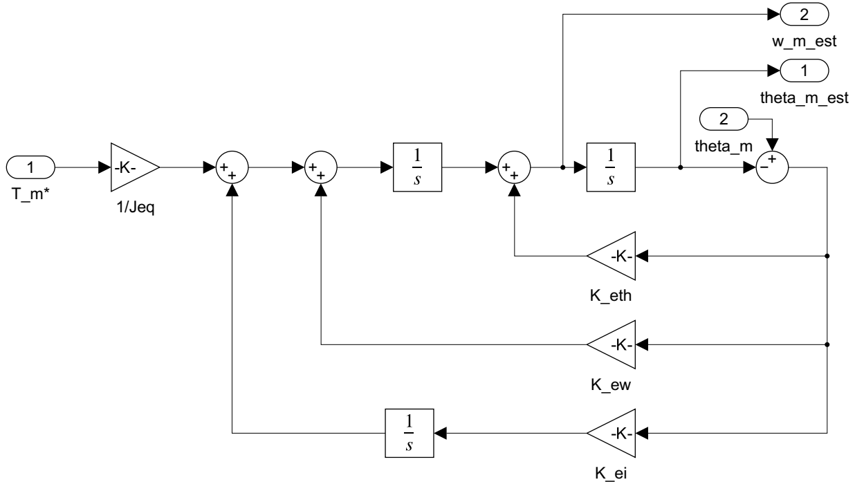
Figura 76: Diagrama de bloques del Observador de Estado Extendido en Simulink. La adición del estado integrador ( K_{ei}/s ) elimina el error de estimación estacionario ante torques de carga desconocidos.
