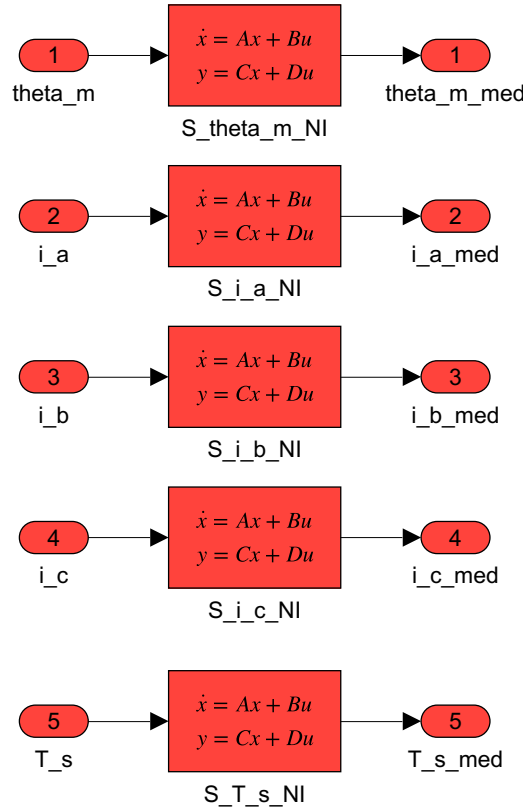
Figura 84: Diagrama de bloques implementado en Simulink para la degradación de los sensores. Cada bloque State-Space se configura con las matrices de diseño y condiciones iniciales rigurosamente calculadas para asegurar un arranque sin transitorios.
