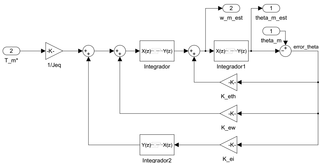
Figura 98: Topología discreta del Observador de Estado Reducido Extendido.
