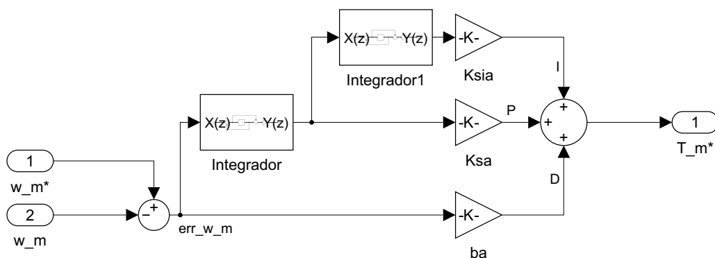
Figura 97: Estructura del Controlador PID en dominio discreto, reemplazando los integradores continuos por equivalentes trapezoidales de Tustin con T_s = 0,0001 s.
