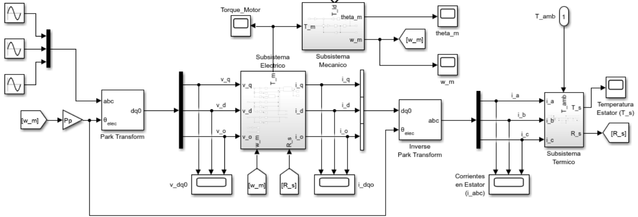
Figura 4: Modelo global no lineal del accionamiento PMSM implementado en Simulink, compuesto por los subsistemas eléctrico, mecánico y térmico, junto con las transformaciones de Park directa e inversa.
