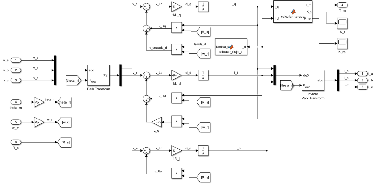
Figura 2: Diagrama de bloques del subsistema electromecánico de la máquina.
