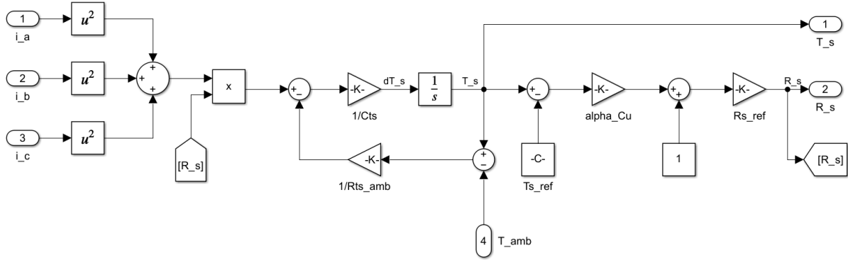
Figura 3: Diagrama de bloques del subsistema térmico de la máquina.
