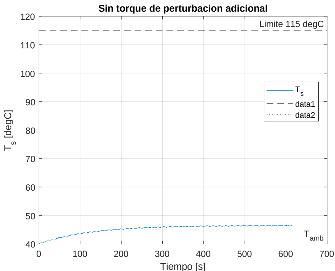
Figura 88: Temperatura del bobinado estático sin torque de perturbacion.
