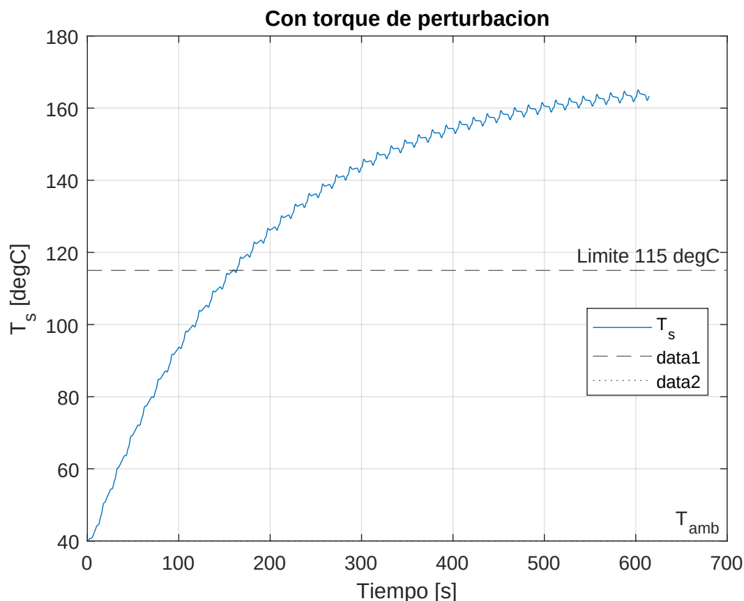
Figura 89: Temperatura del bobinado estático con torque de perturbación sostenido.
