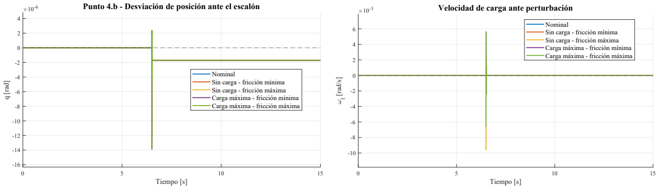
(a) Posición real de la carga para las distintas condiciones mecánicas.
