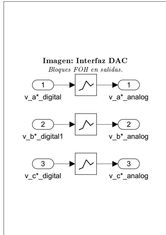
Figura 97: Conversores DAC implementados mediante retención de primer orden (FOH).
