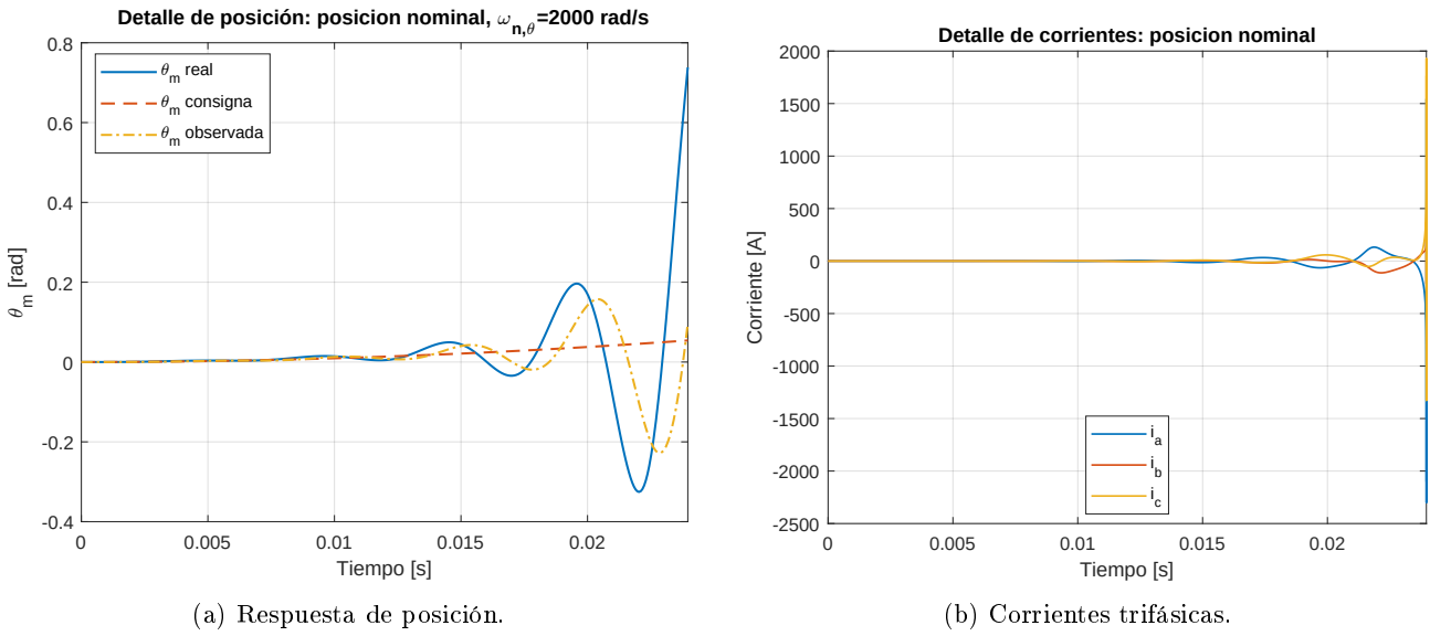
Figura 91: Respuesta del sistema con el sensor de posición nominal, \omega_{n,\theta} = 2000 rad/s: (a) divergencia de la posición real y observada; (b) crecimiento no admisible de las corrientes de fase.
