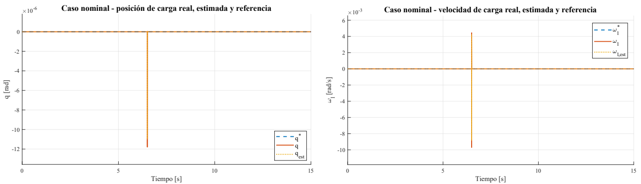
(a) Posición real, estimada y de referencia de la carga.
