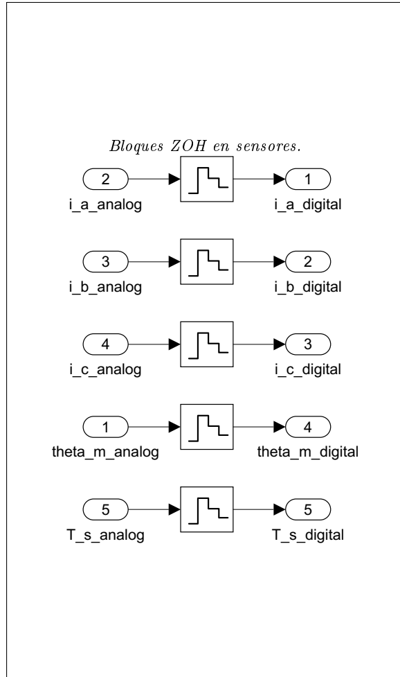
Figura 96: Conversores ADC implementados mediante retención de orden cero (ZOH).
