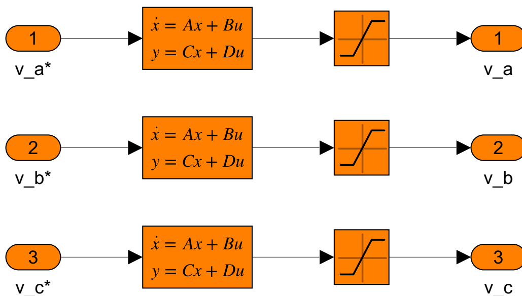
Figura 95: Diagrama de bloques del Modulador Trifásico de Tensión No Ideal en Simulink. A la izquierda se observa la estructura interna por fase incorporando la saturación estricta ( \pm 39,19 V) y la degradación dinámica en Espacio de Estados; a la derecha, el bloque consolidado.
