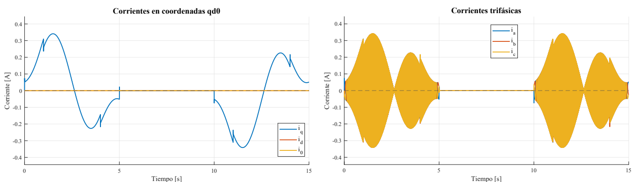
(a) Corrientes en coordenadas qd0 .
