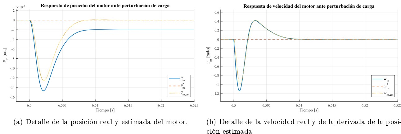
Figura 72: Detalle de la respuesta del motor en el instante de aplicación de la perturbación para el caso nominal. La velocidad retorna a cero, mientras que la posición conserva una pequeña desviación estacionaria.
