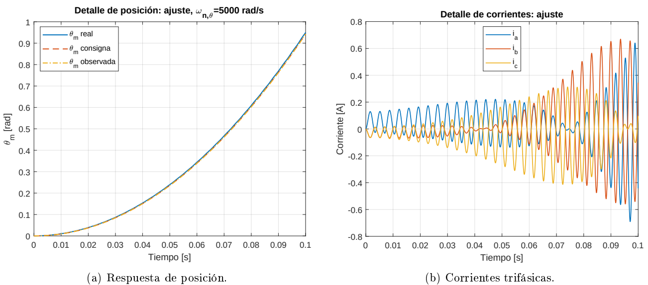
Figura 92: Respuesta del sistema con el sensor de posición ajustado a \omega_{n,\theta} = 5000 rad/s: (a) seguimiento adecuado de posición; (b) oscilaciones todavía presentes en las corrientes de fase.
