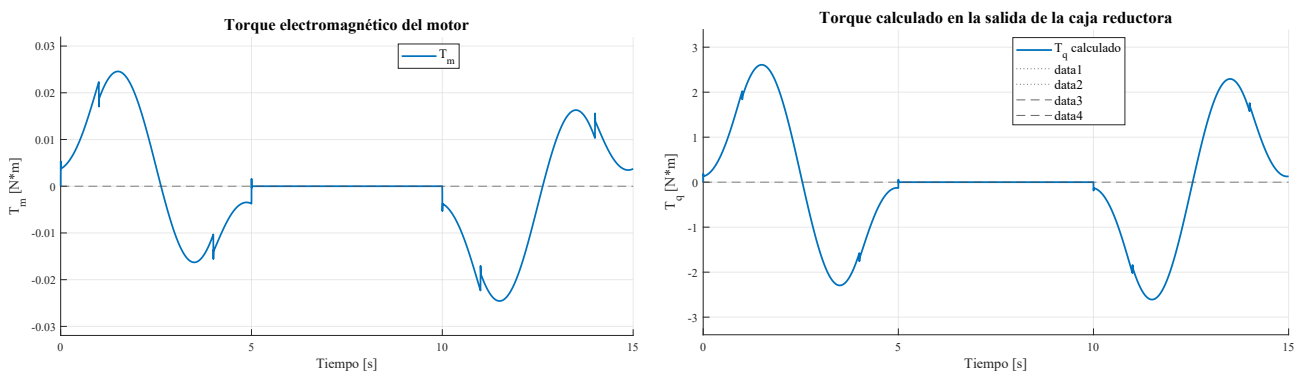
(a) Torque electromagnético desarrollado por el motor.
