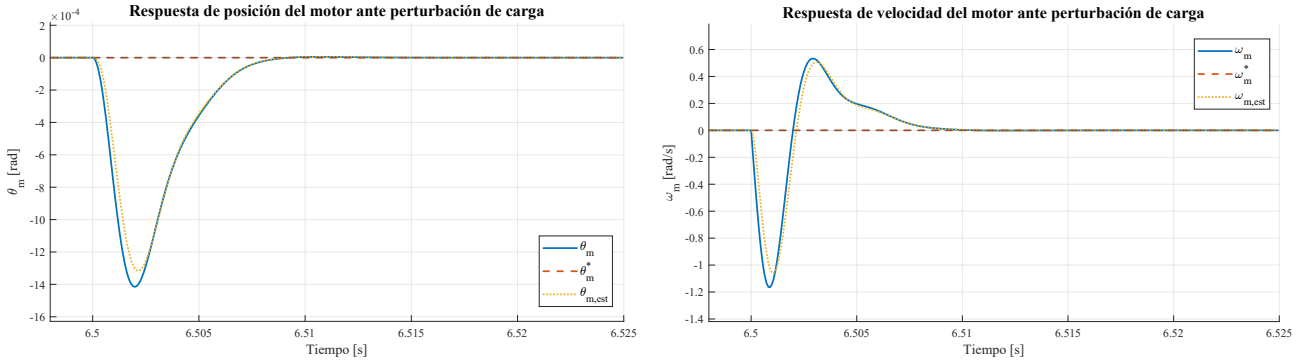
(a) Detalle de la posición real y estimada del motor.
