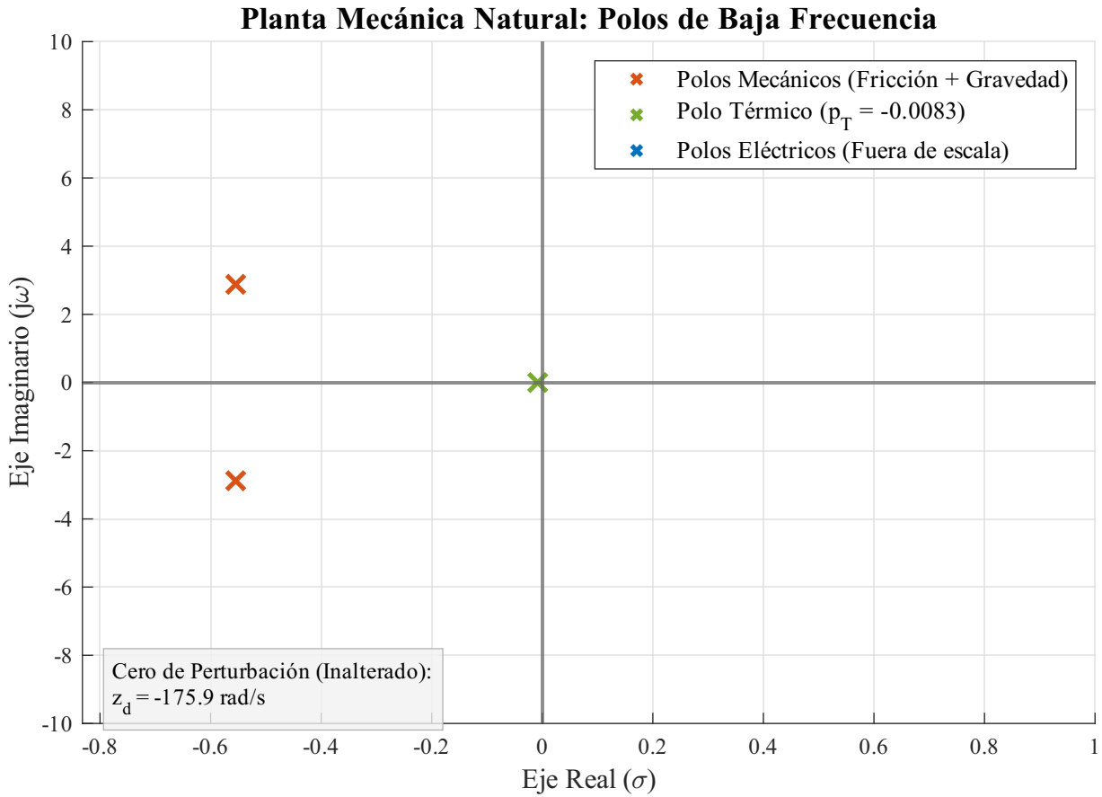
Figura 48: Detalle de los polos del sistema mecánico natural a baja frecuencia. La fricción viscosa y el torque gravitacional desvían la dinámica respecto a la de una inercia pura.
