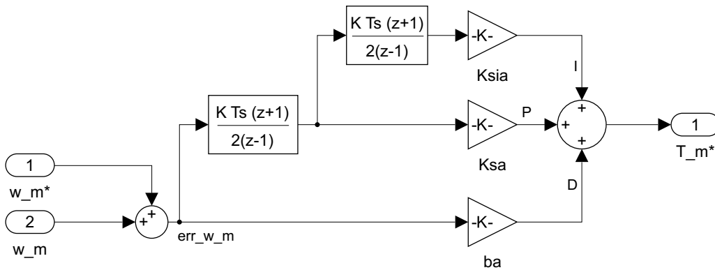
Figura 98: Estructura del Controlador PID en dominio discreto, reemplazando los integradores continuos por equivalentes trapezoidales de Tustin con T_s = 0,0001 s.
