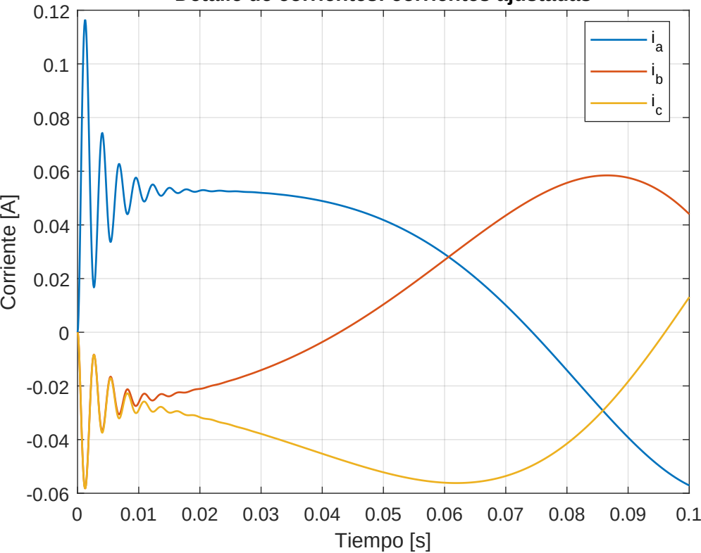
Detalle de corrientes: corrientes ajustadas
