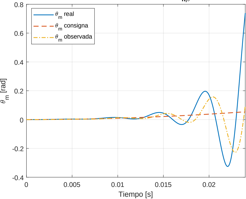
Detalle de posición: posición nominal, \omega_{n,\theta}=2000 rad/s
