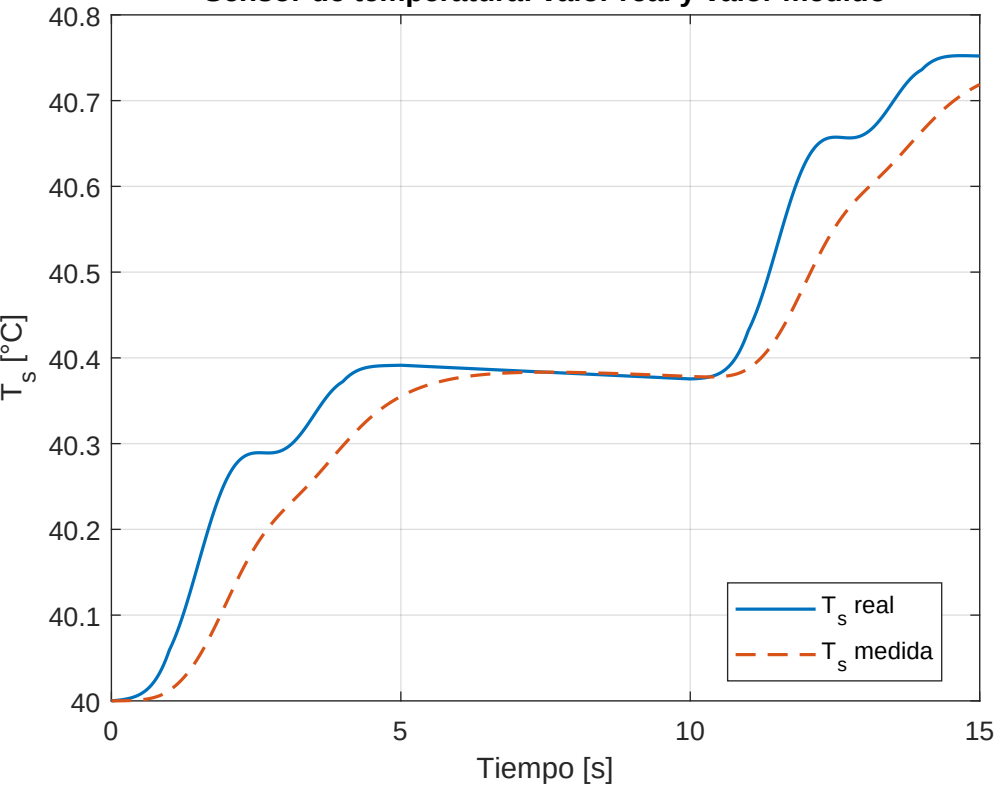
Sensor de temperatura: valor real y valor medido
