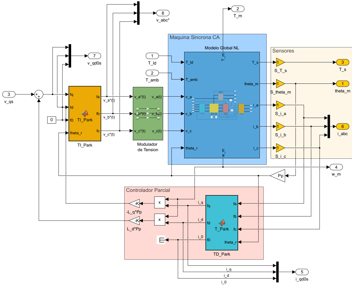
Figura 9: Implementación de la ley complementaria mínima en el eje q para cancelar el acoplamiento no lineal residual producido por i_{ds}^r(t) .
