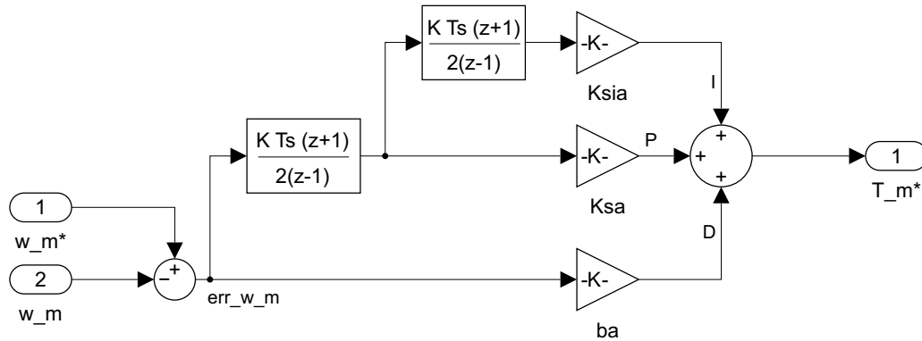
Figura 101: Estructura del Controlador PID en dominio discreto, reemplazando los integradores continuos por equivalentes trapezoidales de Tustin con T_s = 0,0001 s.
