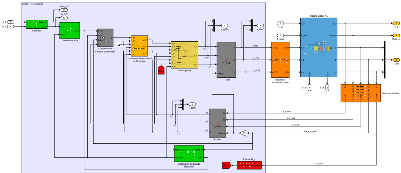
Figura 65: Diagrama Sistema de Control completo.
