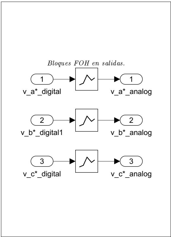
Figura 100: Conversores DAC implementados mediante retención de primer orden (FOH).
