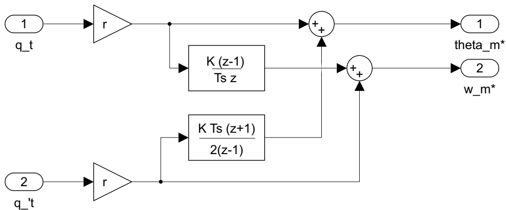
Figura 103: Implementación en tiempo discreto de la Interfaz de Referencia (Set-Point).
