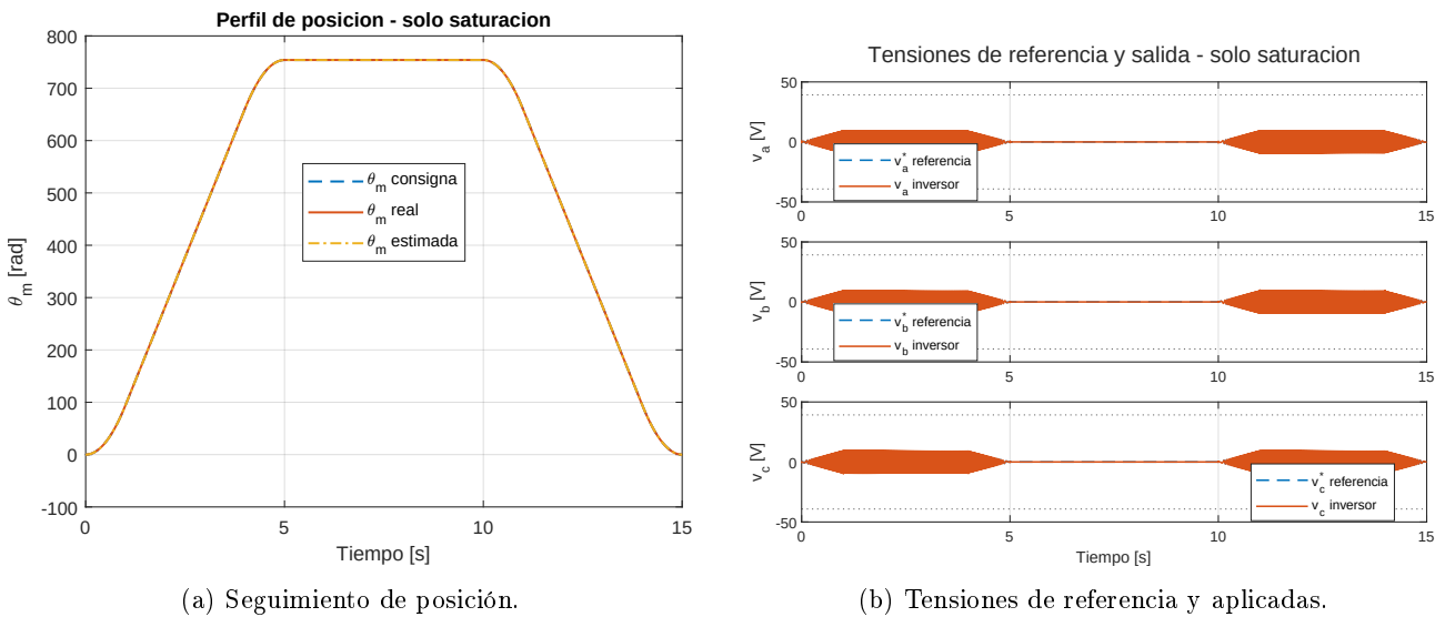
Figura 96: Respuesta considerando únicamente la saturación del inversor.
