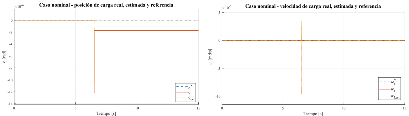
(a) Posición real, estimada y de referencia de la carga. (b) Velocidad real, señal de realimentación y referencia de la carga.
