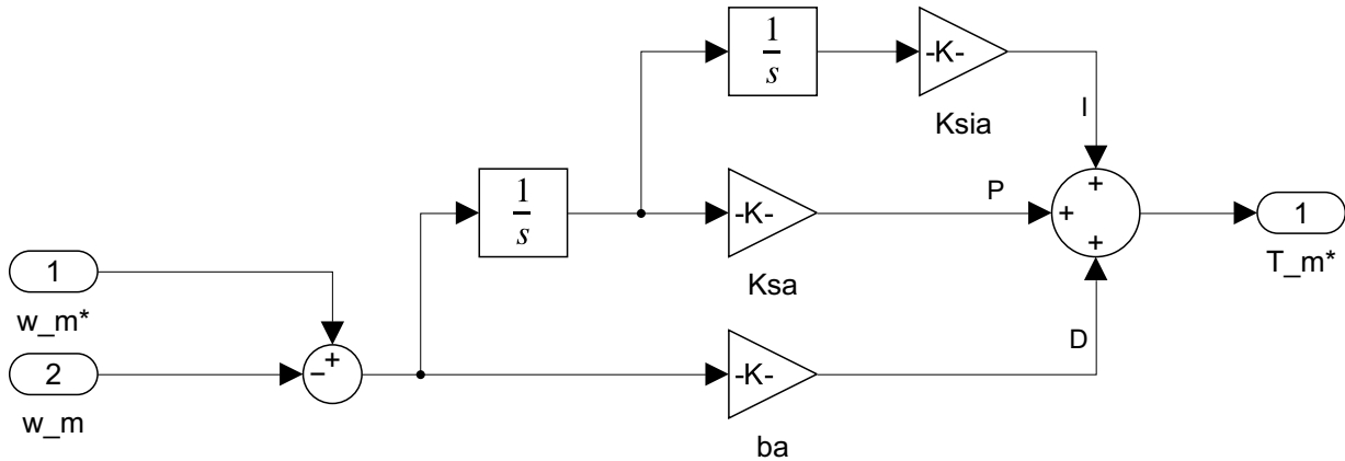
Figura 58: Implementación del controlador PID de movimiento en Simulink. La estructura utiliza integradores en cascada y una consigna de velocidad intermedia para evitar el uso de derivadores puros.
