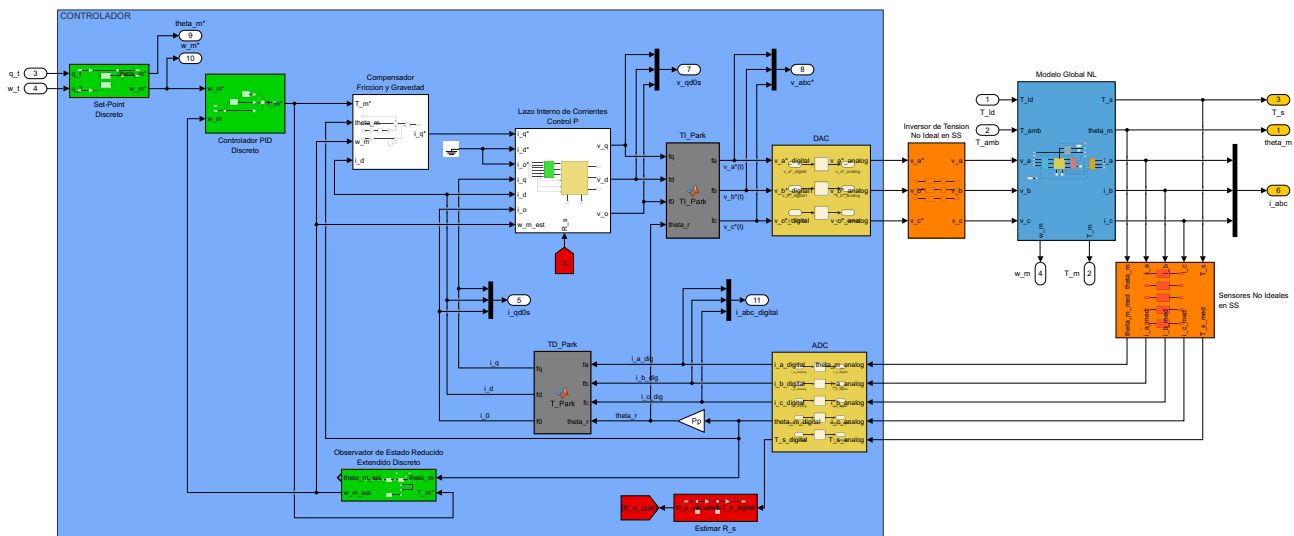
Figura 104: Arquitectura integral del controlador en cascada discretizado.
