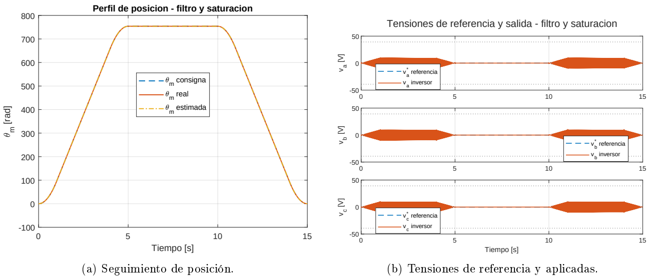
Figura 98: Respuesta del inversor completo para \omega_{n,v} = 27000 rad/s.
