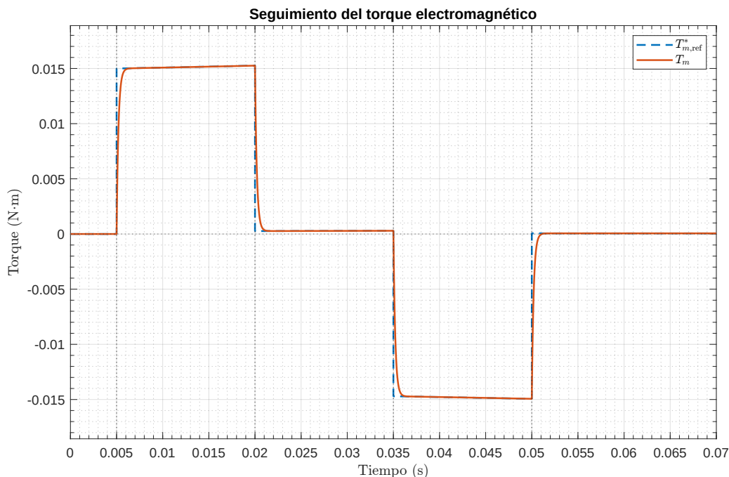
Figura 53: Seguimiento de la referencia electromagnética total por el torque generado por la máquina.
