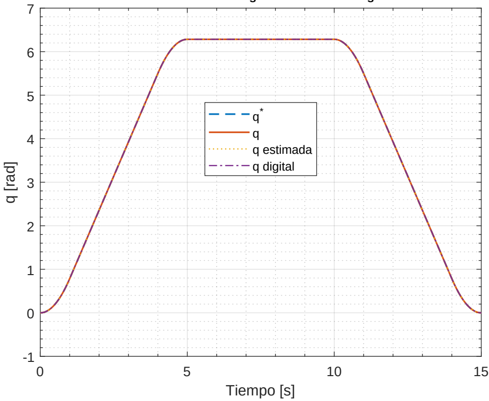
Seguimiento de posición - f_s = 10.000 \text{ kHz} , T_s = 100.000 \text{ us}
