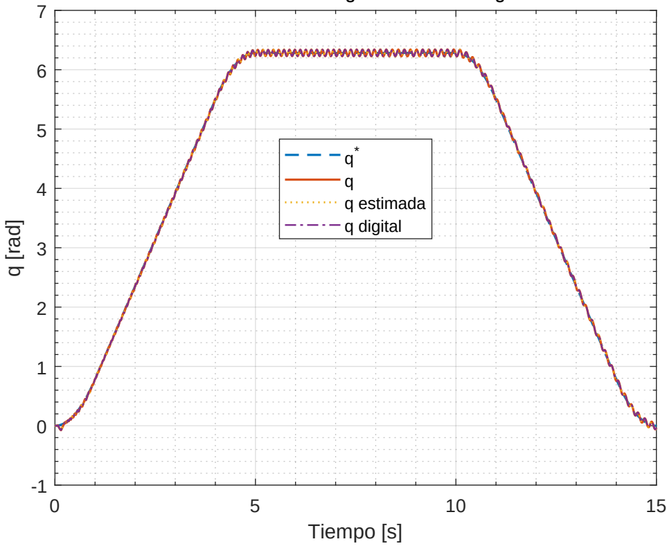
Seguimiento de posición - f_s = 5.000 kHz, T_s = 200.000 us
