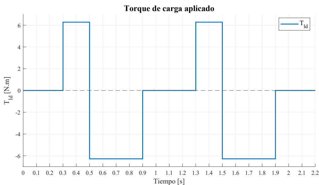
Figura 15: Perturbación de torque de carga aplicada al sistema, T_{ld}(t) .
