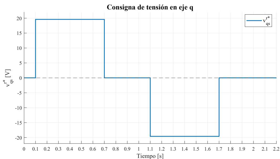
Figura 14: Consigna de tensión aplicada en el eje q , v_{qs}^r(t) .
