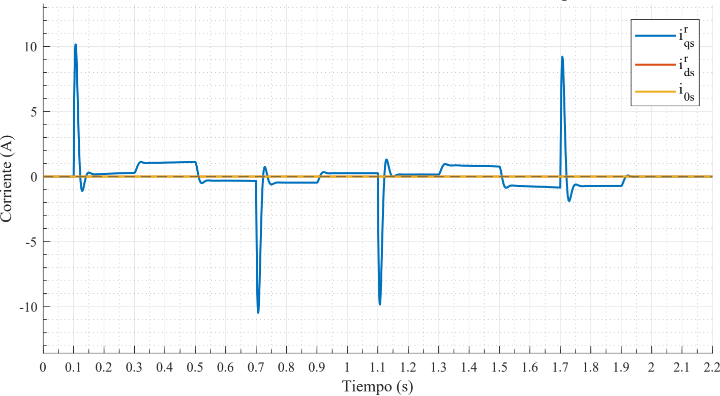
Corrientes del modelo no lineal en coordenadas qd0
