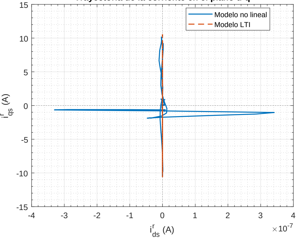
Trayectoria de la corriente en el plano d-q
