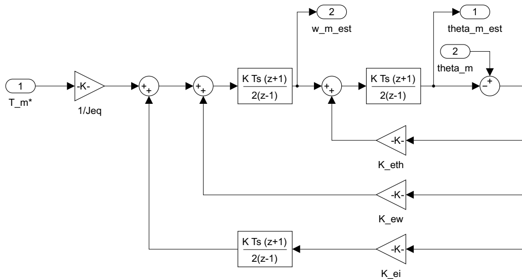
Figura 99: Topología discreta del Observador Reducido de Estado, forzando la digitalización de sus entradas y su dinámica interna mediante el método bilineal.
