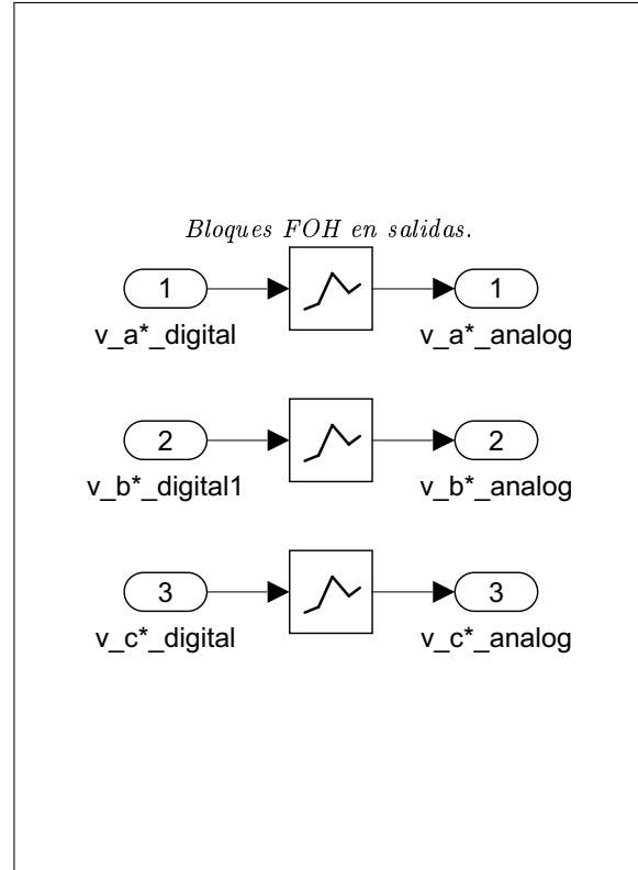
Figura 97: Conversores DAC implementados mediante retención de primer orden (FOH).
