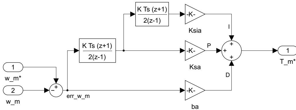
Figura 98: Estructura del Controlador PID en dominio discreto, reemplazando los integradores continuos por equivalentes trapezoidales de Tustin con T_s = 0,0001 s.
