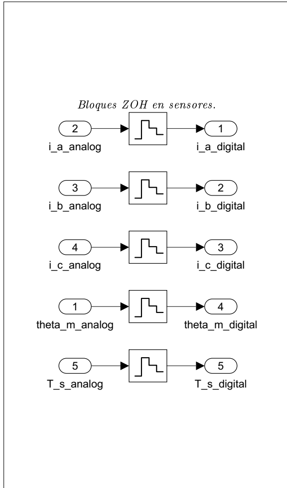
Figura 96: Conversores ADC implementados mediante retención de orden cero (ZOH).
