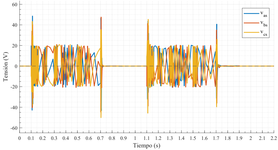
Figura 25: Tensiones estadóricas de fase v_a(t) , v_b(t) y v_c(t) , expresadas en coordenadas abc .
