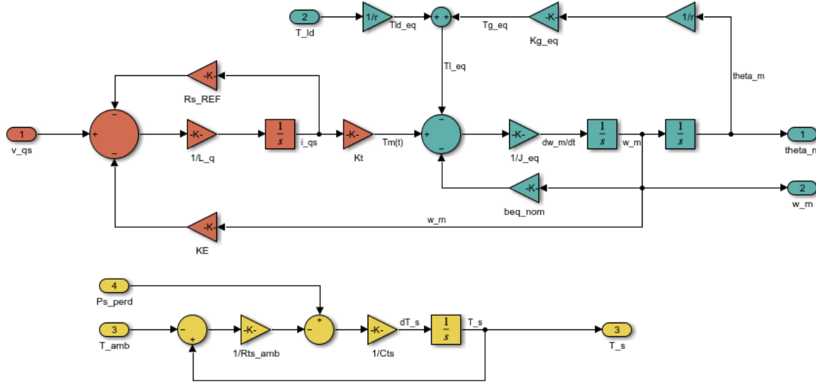
Figura 5: Diagrama de bloques del modelo LTI electromecánico equivalente por realimentación no lineal. Se muestra la dinámica principal de tres estados v_{qs}^r(t) \rightarrow i_{qs}^r(t) \rightarrow T_m(t) \rightarrow \omega_m(t) \rightarrow \theta_m(t) , junto con la perturbación mecánica externa, la gravedad linealizada y la rama térmica auxiliar excitada por P_{s,perd}(t) .
