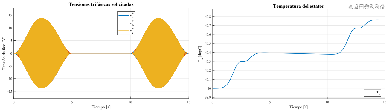
Figura 80: Tensiones solicitadas y respuesta térmica para el perfil polinómico de quinto orden.
